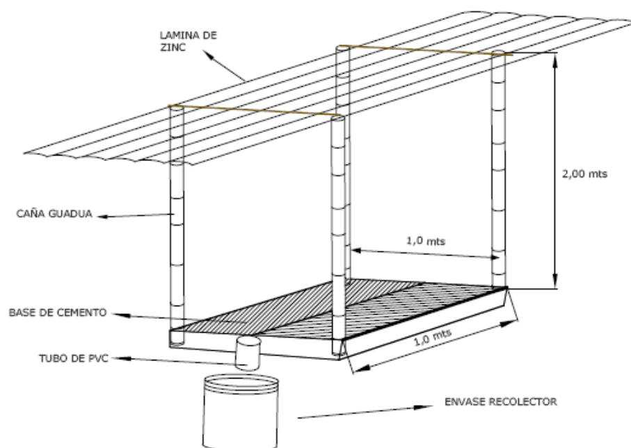
FIGURA 3.1. INFRAESTRUCTURA LIXIVIADORES.
