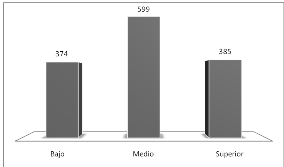
GRAFICO 6. REPRESENTACION GRAFICA DE LA ABUNDANCIA DEL TOTAL DE INDIVIDUOS EN LOS DIFERENTES ESTRATOS.
