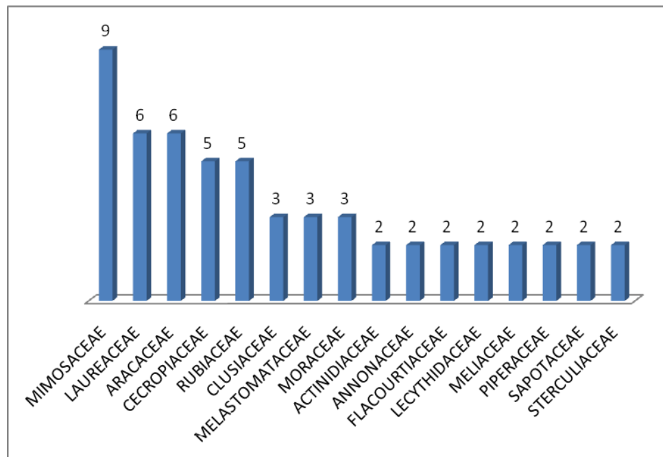
GRAFICO 2. ABUNDANCIA DE ESPECIES POR FAMILIA BOTANICA.
