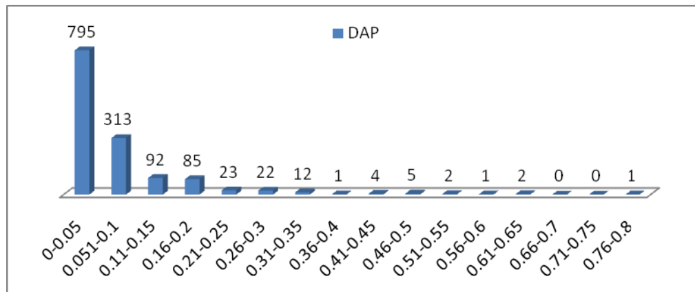
GRAFICO 9. DISTRIBUCION DIAMETRICA DE LOS INDIVIDUOS MUESTREADOS.
