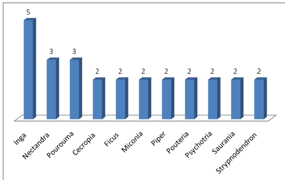
GRAFICO 3. ABUNDANCIA DE ESPECIES POR GENERO BOTANICO.
