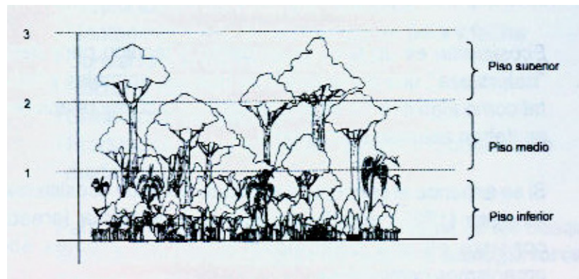
FIGURA 1.2.2. ESTRUCTURA VERTICAL DEL BOSQUE SEGÚN IUFRO.
