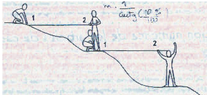
FIGURA 2.5.2. MEDICIÓN DE DISTANCIAS HORIZONTALES EN PENDIENTE.
