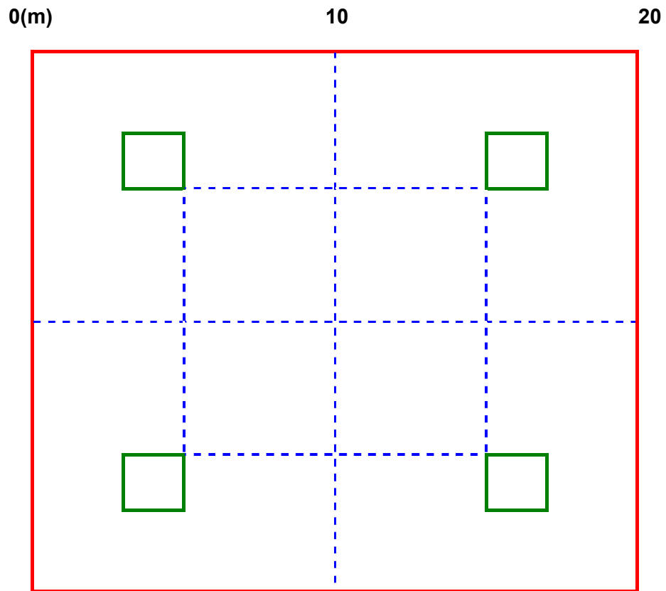
FIGURA 3.3.1. DISEÑO DE LA UNIDAD DE MUESTREO.
