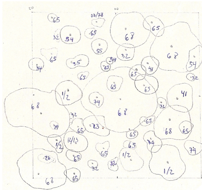
GRAFICO 21. ESTRUCTURA HORIZONTAL DEL BOSQUE PERTURBADO.
