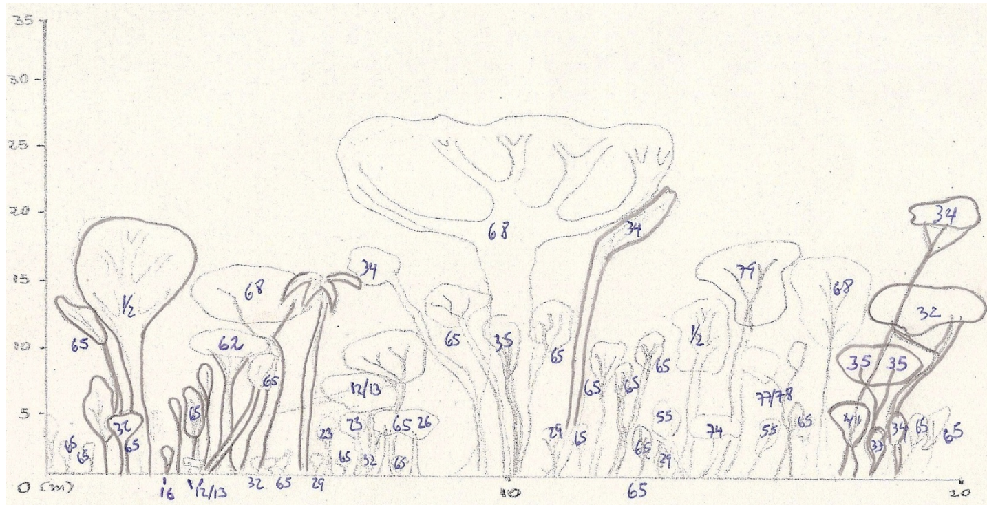
GRAFICO 22. ESTRUCTURA VERTICAL DEL BOSQUE PERTURBADO.
