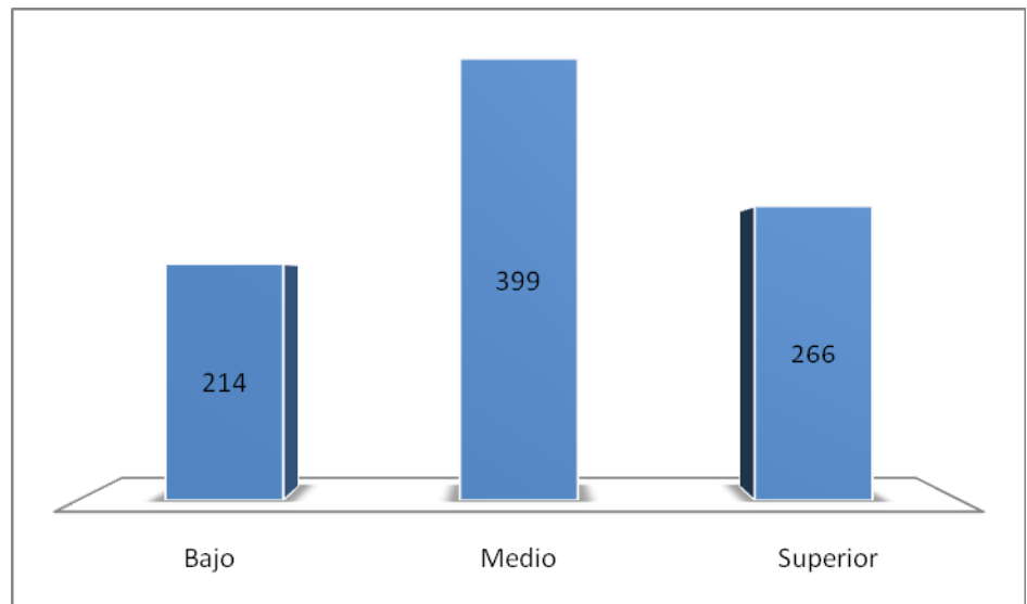
GRAFICO 7. REPRESENTACION GRAFICA DE LA ABUNDANCIA DE ESPECIES MAS REPRESENTATIVAS EN LOS DIFERENTES ESTRATOS.
