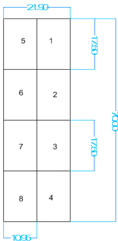
FIGURA 4.9: ESPACIO DISPONIBLE PARA ASIGNACIÓN DE DEPARTAMENTOS
