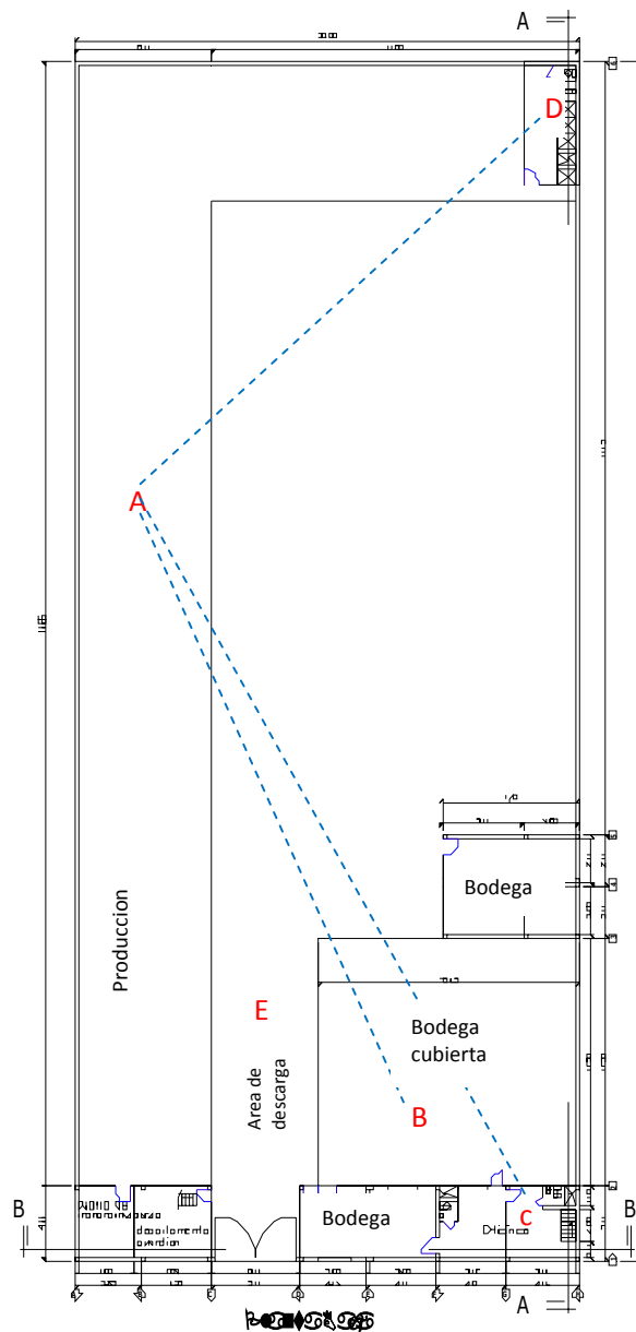
PLANO 1: DISTRIBUCIÓN ACTUAL DE LA PLANTA
