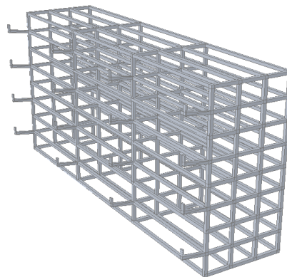
FIGURA 3.17 ESTRUCTURA DE SOPORTE PARA TUBOS
