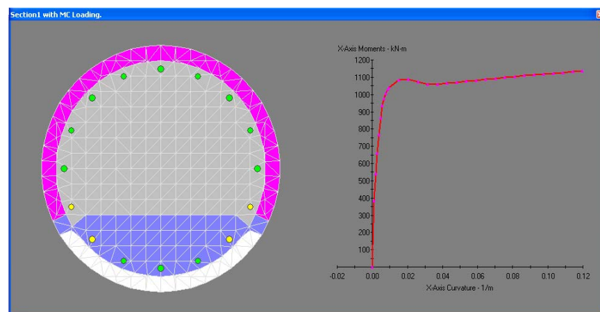
Figura 4.40: Resultado del Análisis Momento Curvatura.
