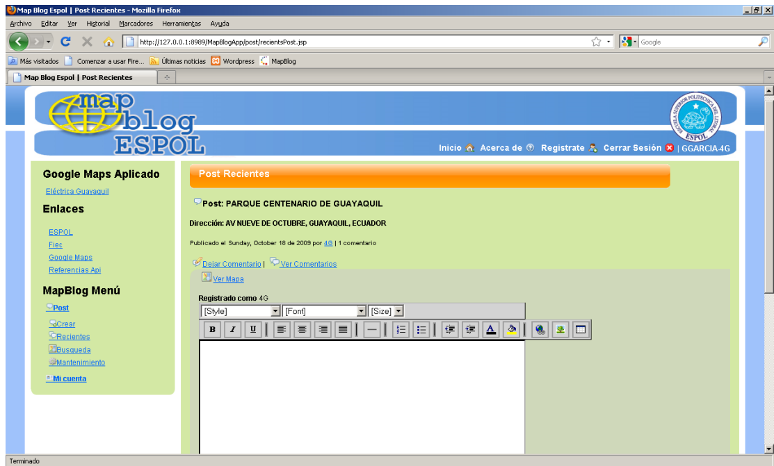
Figura 2-12 Entradas Recientes
