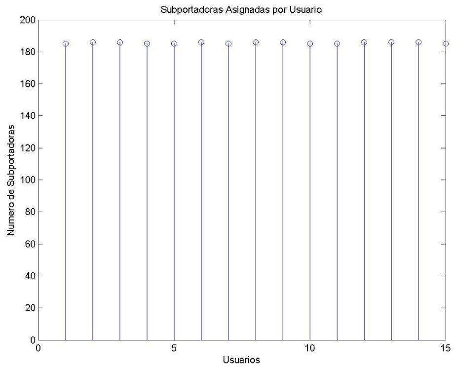
Fig. 5 Esquema de asignación de bits para 15 usuarios a 500 m.
