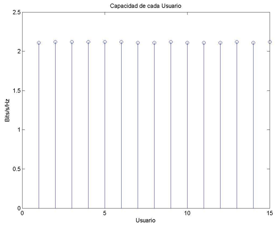
Fig. 16 Bits asignados por usuario cuando se tienen 15 usuarios a 1500 m
