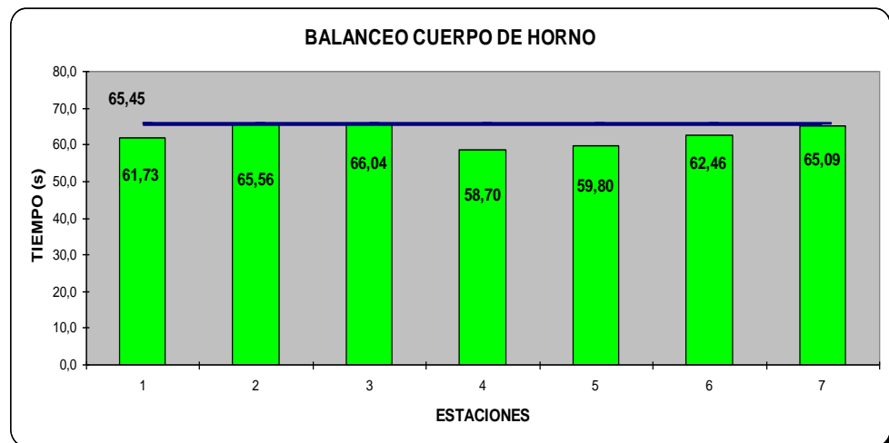
FIGURA 4.14, BALANCEO CUERPO DE HORNO
