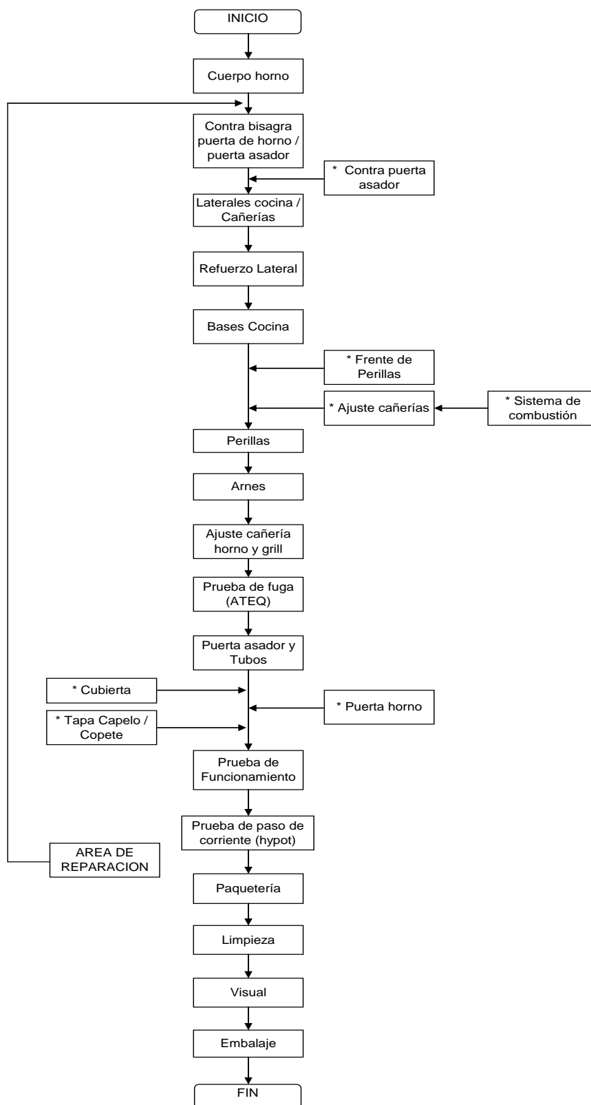
FIGURA 3.5 SECUENCIA DE OPERACIONES PARA LAS COCINAS DE 20", 24" Y 35".
