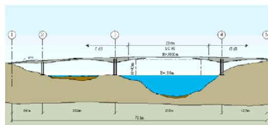
Figura 2. Esquema de ubicación de secciones postensadas de HLAD
