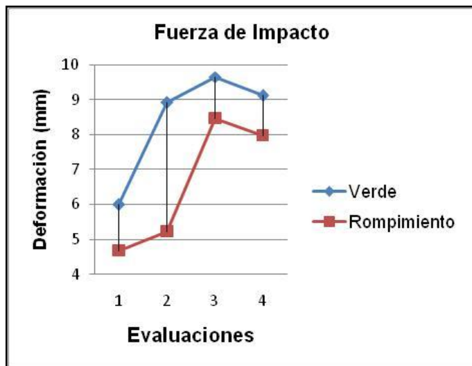
FIGURA 3.24 B COMPORTAMIENTO DE LA DEFORMACIÓN EN FUNCIÓN DEL TIEMPO-FUERZA DE IMPACTO Elaborado por: Jonathan Coronel León
