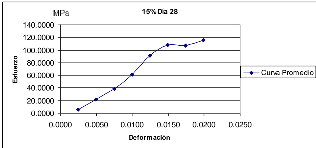
Figura 4.2. Curva esfuerzo-deformación
