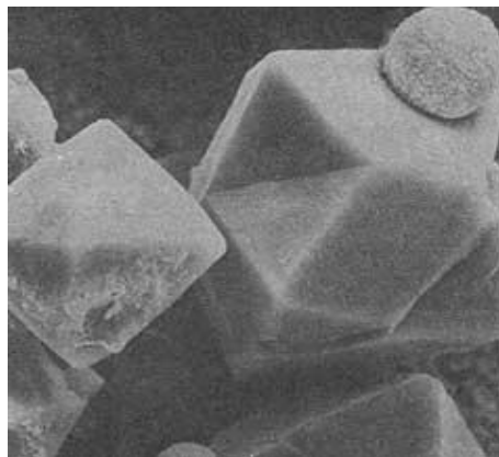
Figura 2.3. Zeolita faujasita. Observada en el microscopio electrónico de barrido. Los cristales son de 50 Å aproximadamente.
