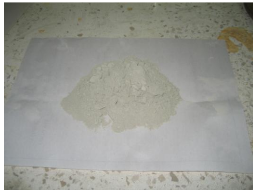
Figura 3.10. Tamizado y zeolita final
