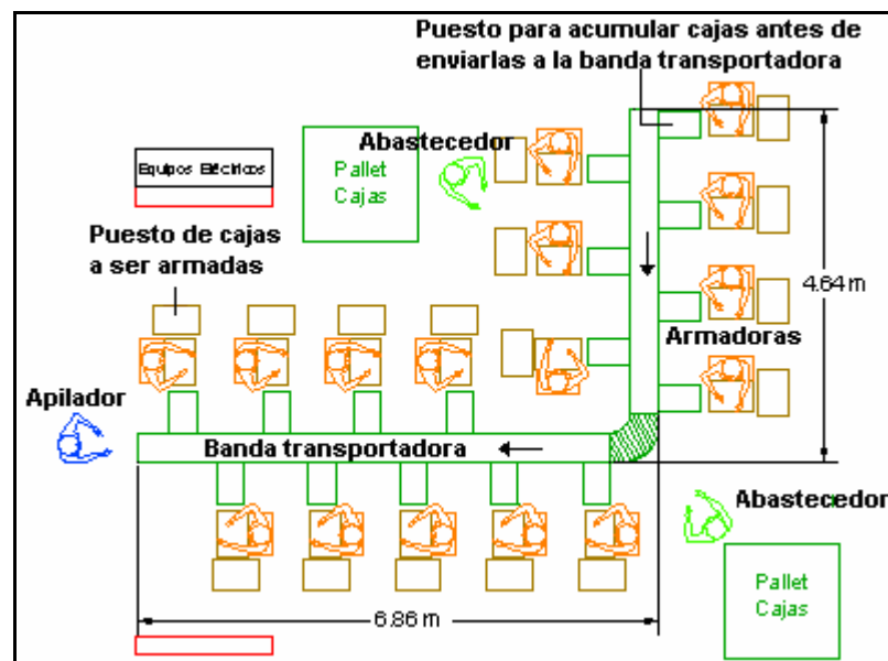
FIGURA 4.6 ARREGLO DE LAS ARMADORAS MANUALES DE CAJAS ALREDEDOR DE UNA BANDA TRANSPORTADORA EN L
