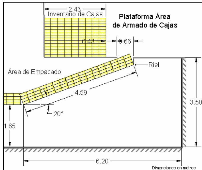
FIGURA 5.4 DIMENSIONES DE LOS RIELES PROPUESTOS CON INCLINACIÓN DE 20°
