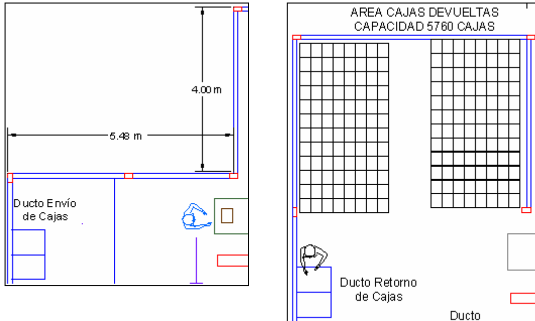
FIGURA 6.5 SITUACIÓN ACTUAL Y PROPUESTA PARA EL DESARROLLO DEL ÁREA DE CAJAS DEVUELTAS
