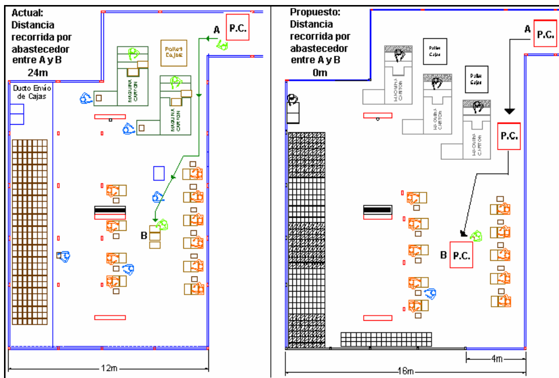
FIGURA 6.1 AMPLIACIÓN DE LA PLATAFORMA DEL ÁREA DE ARMADO DE CAJAS
