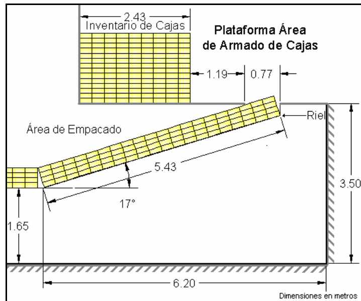
FIGURA 5.6 DIMENSIONES DE LOS RIELES PROPUESTOS CON INCLINACIÓN DE 17°
