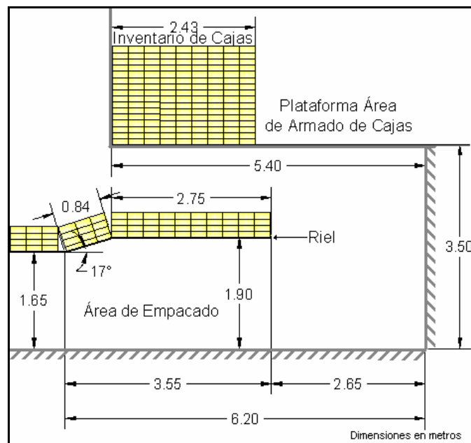
FIGURA 5.3 DIMENSIONES DE LOS RIELES ACTUALES
