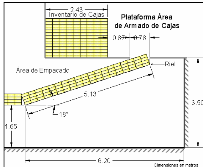
FIGURA 5.5 DIMENSIONES DE LOS RIELES PROPUESTOS CON INCLINACIÓN DE 18°
