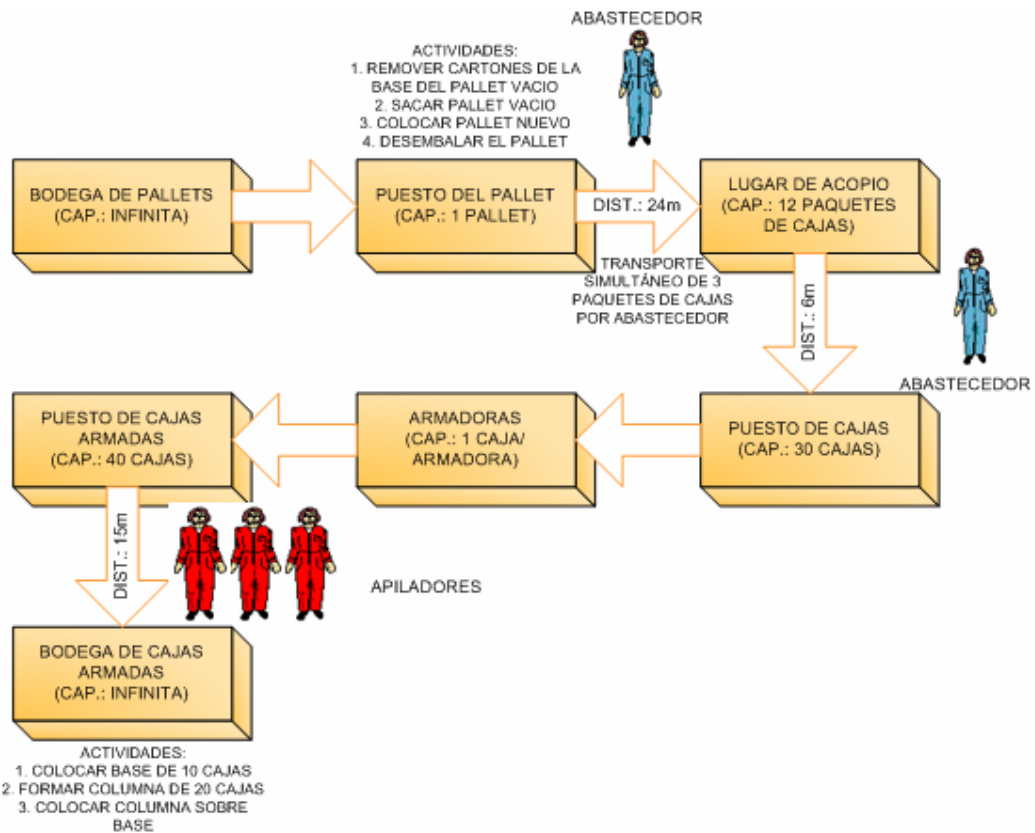
FIGURA 3.1 SECUENCIA DE LAS ACTIVIDADES PARA EL ARMADO MANUAL DE CAJAS
