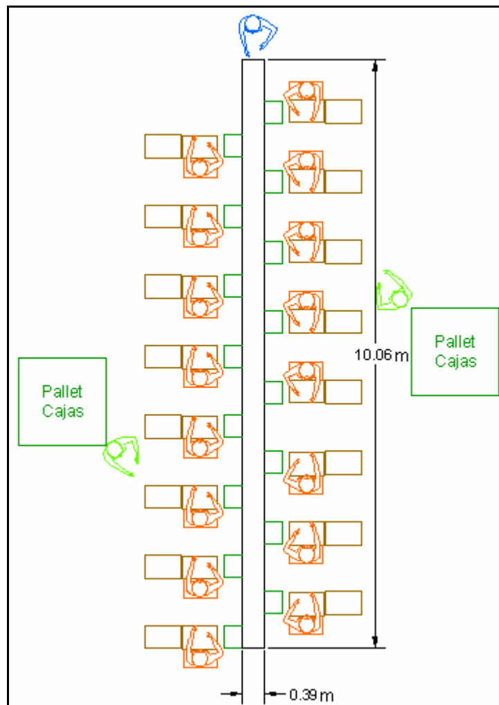
FIGURA 4.7 ARREGLO DE LAS ARMADORAS MANUALES DE CAJAS ALREDEDOR DE UNA BANDA TRANSPORTADORA EN LÍNEA RECTA
