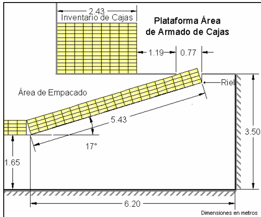
FIGURA 6.3 DIMENSIONES DE LOS RIELES QUE CONECTAN EL ÁREA DE ARMADO DE CAJAS CON EL ÁREA DE EMPACADO
