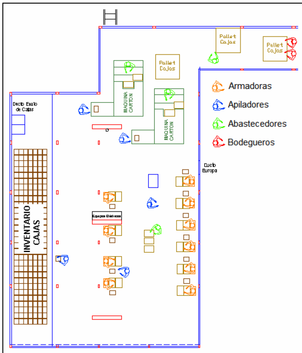
FIGURA 2.13 PLATAFORMA DEL ÁREA DE ARMADO DE CAJAS
