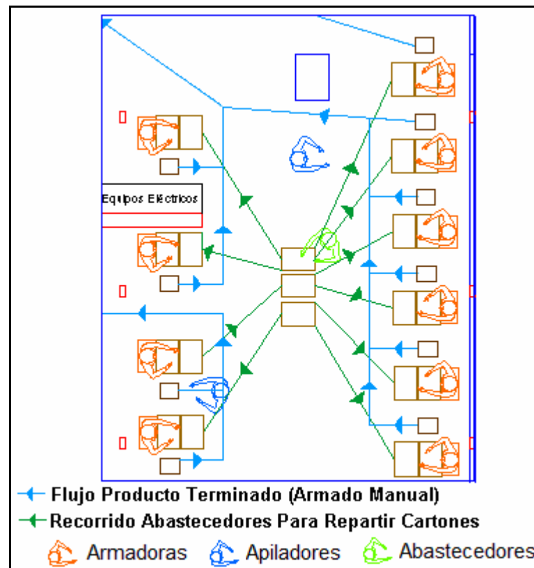
FIGURA 4.1 DIAGRAMA DE FLUJO DEL ABASTECIMIENTO DE CAJAS PARA ARMADO MANUAL Y RECOLECCIÓN DEL PRODUCTO TERMINADO
