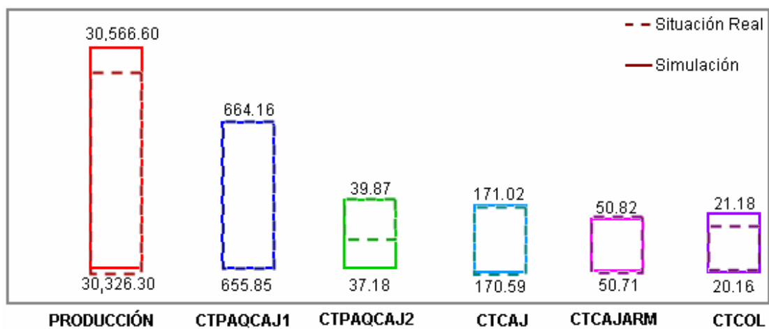
FIGURA 3.7 COMPARACIÓN DE LOS INTERVALOS DE CONFIANZA DE LOS PARÁMETROS
