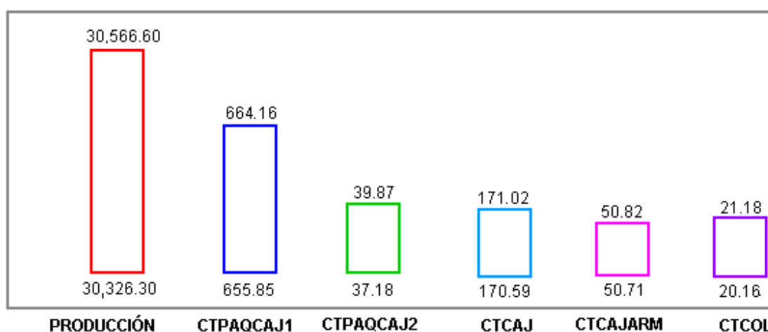
FIGURA 3.6 INTERVALOS DE CONFIANZA DE LOS PARÁMETROS DE VALIDACIÓN DEL MODELO DE SIMULACIÓN
