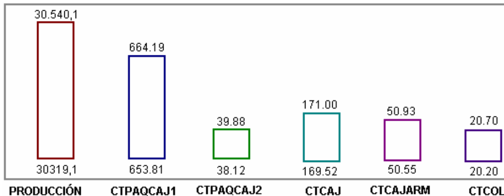
FIGURA 3.5 INTERVALOS DE 95% DECONFIANZA DE LOS PARÁMETROS DE COMPARACIÓN
