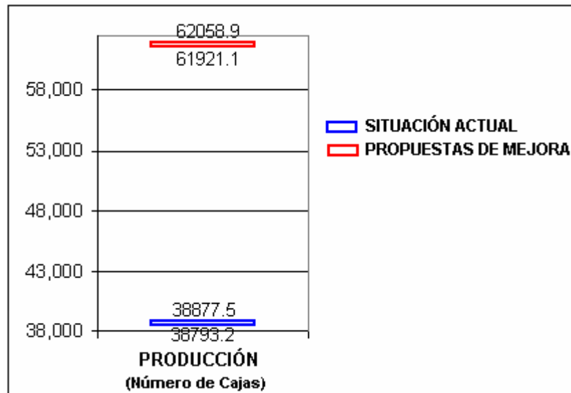
FIGURA 4.16 INTERVALO DE CONFIANZA DE LA PRODUCCIÓN DE LA SIMULACIÓN DE LA SITUACIÓN ACTUAL Y CON LAS MEJORAS
