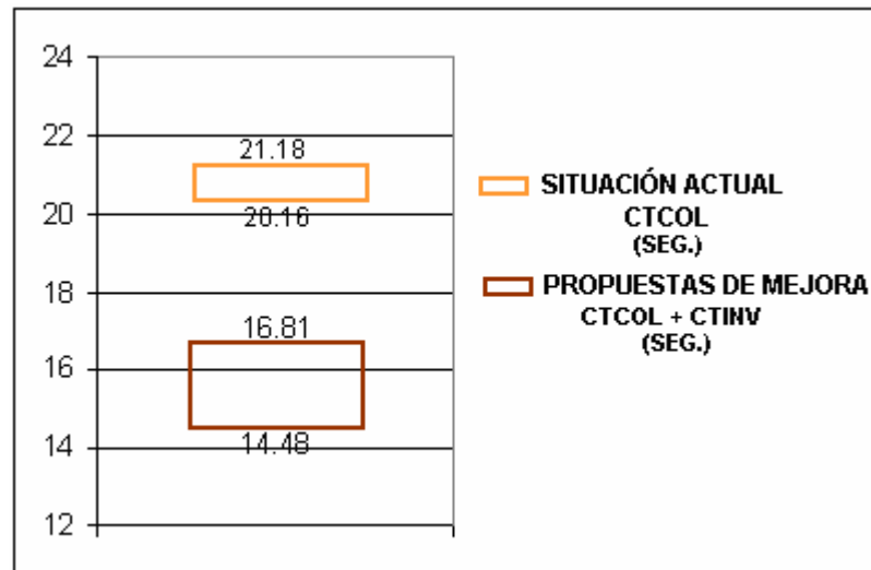
FIGURA 4.14 INTERVALOS DE CONFIANZA DE LOS PARÁMETROS CTCOL Y CTINV
