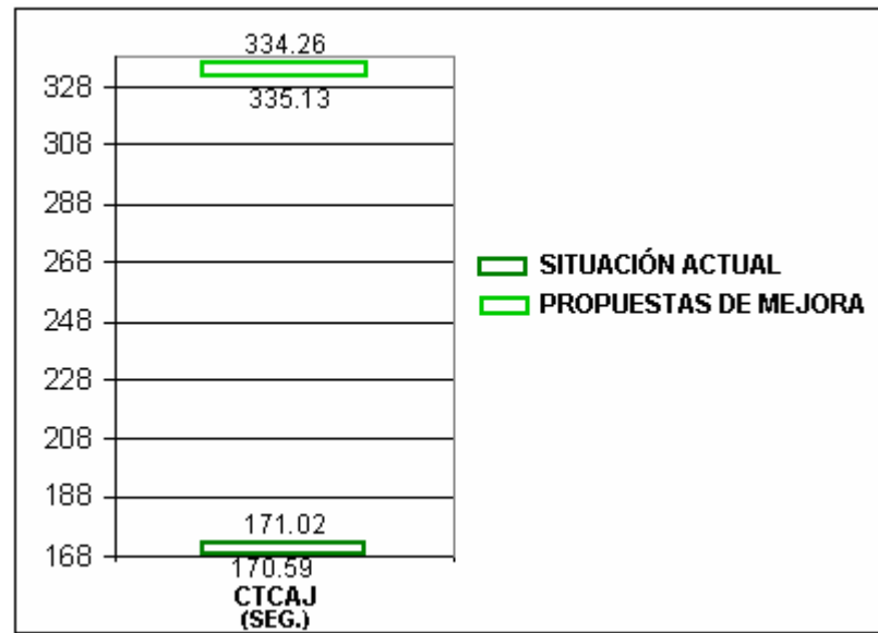
FIGURA 4.12 INTERVALOS DE CONFIANZA PARA EL PARÁMETRO CTCAJ
