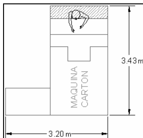
FIGURA 4.4 MÁQUINA ARMADORA DE CAJAS
