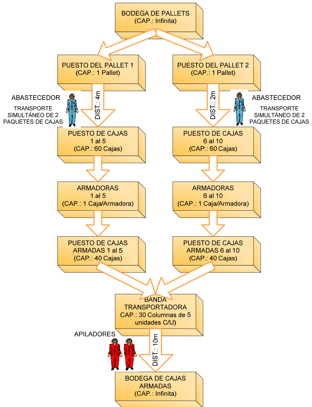
FIGURA 4.8 SECUENCIA DE LAS ACTIVIDADES PARA LA MEJORA PROPUESTA DEL ARMADO MANUAL DE CAJAS
