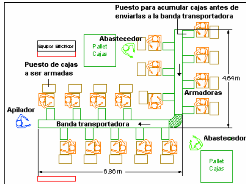
FIGURA 6.2 ARREGLO DE LAS ARMADORAS MANUALES DE CAJAS ALREDEDOR DE UNA BANDA TRANSPORTADORA EN L
