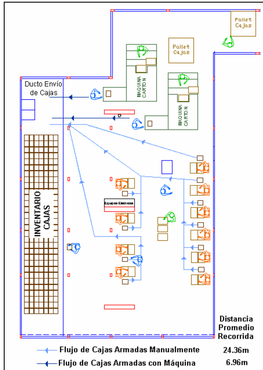
FIGURA 2.15 FLUJO DE CAJAS ARMADAS PARA USO INMEDIATO EN EL ÁREA DE EMPACADO
