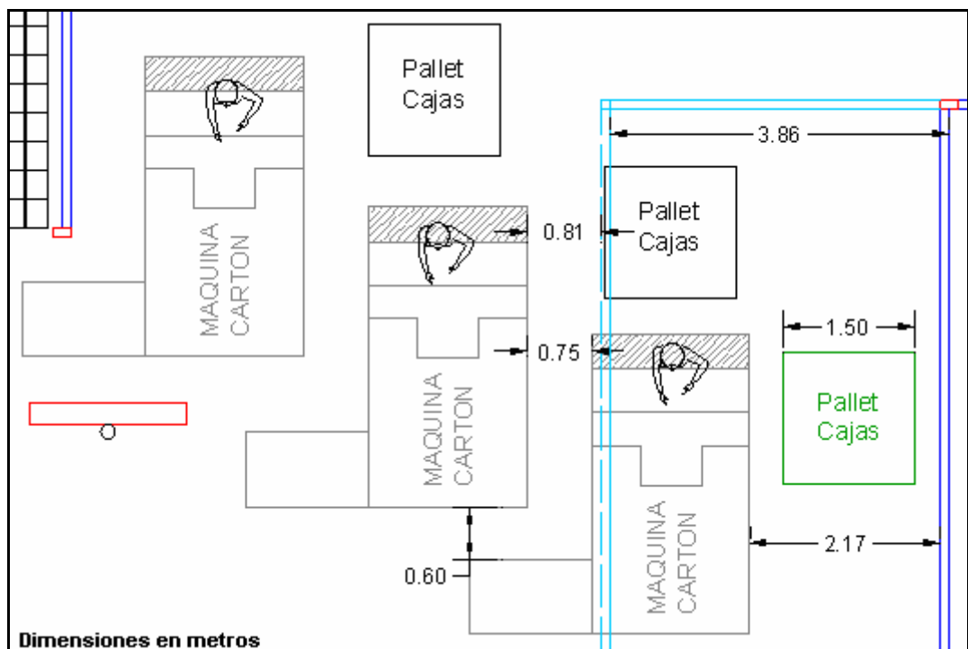
FIGURA 4.5 AMPLIACIÓN DE LA PLATAFORMA DEL ÁREA DE ARMADO DE CAJAS
