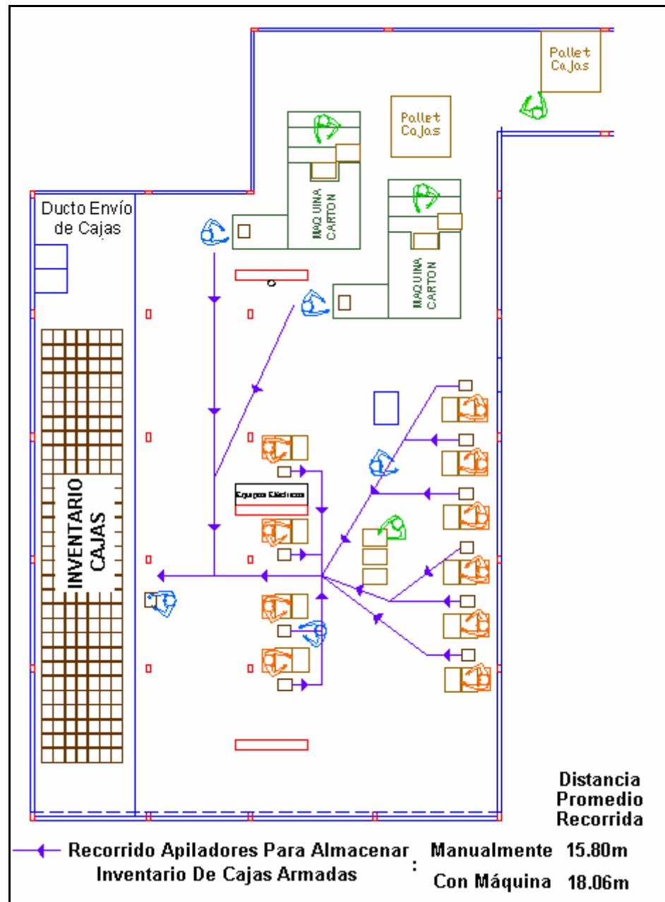
FIGURA 2.16 RECORRIDO DE LOS APILADORES PARA ALMACENAR LAS CAJAS ARMADAS PARA INVENTARIO
