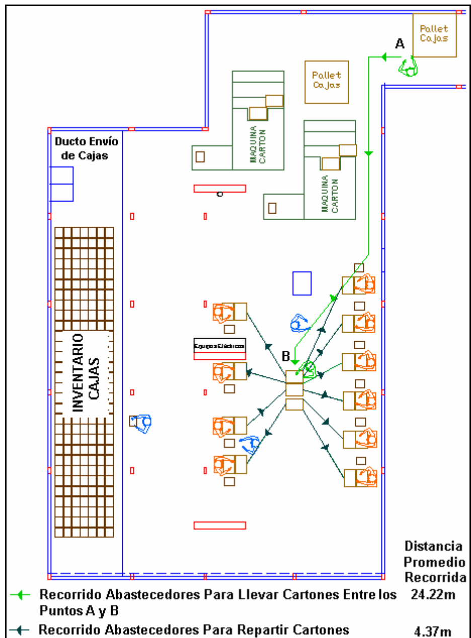
FIGURA 2.14 RECORRIDO DE LOS ABASTECEDORES DE CAJAS
