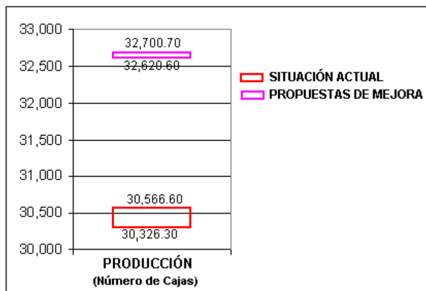
FIGURA 4.15 INTERVALO DE CONFIANZA DE LA VARIABLE PRODUCCIÓN
