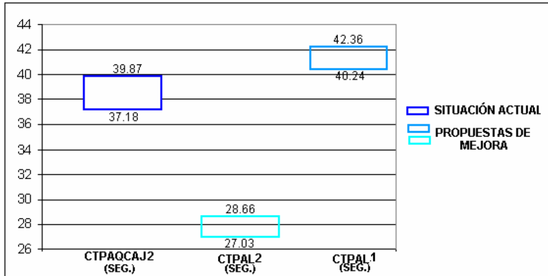
FIGURA 4.11 INTERVALOS DE CONFIANZA DEL PARÁMETRO CTPAL
