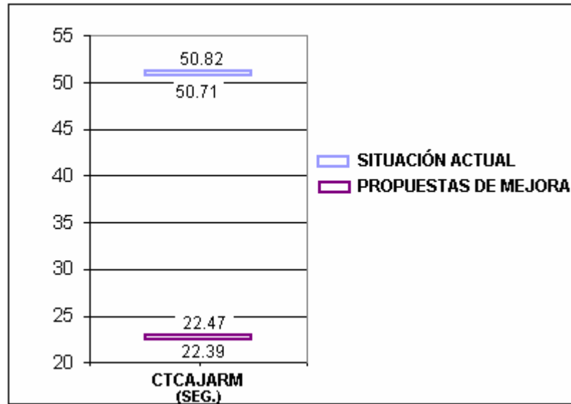
FIGURA 4.13 INTERVALOS DE CONFIANZA PARA EL PARÁMETRO CTCAJARM
