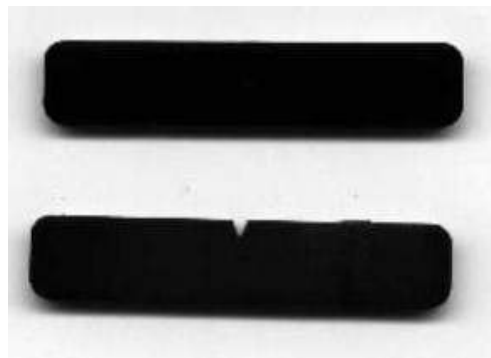
FIGURA 4.5 MUESTRAS DEL ENSAYO IZOD
