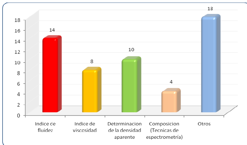
FIGURA 3.2 ENSAYOS REALIZADOS A LA MATERIA PRIMA
