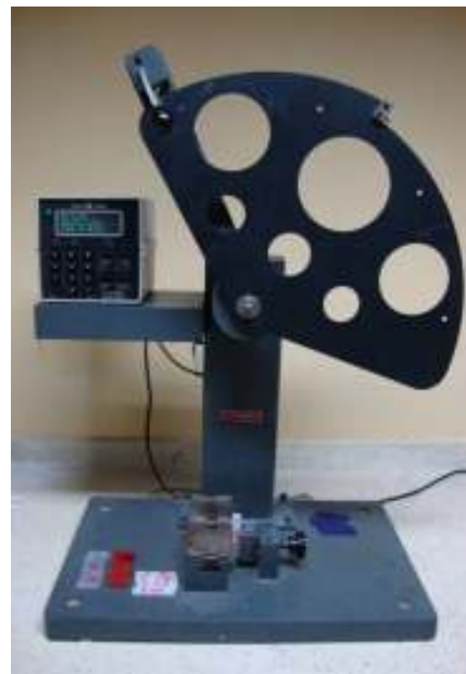
FIGURA 4.4 EQUIPO DE ENSAYO DE IMPACTO IZOD
