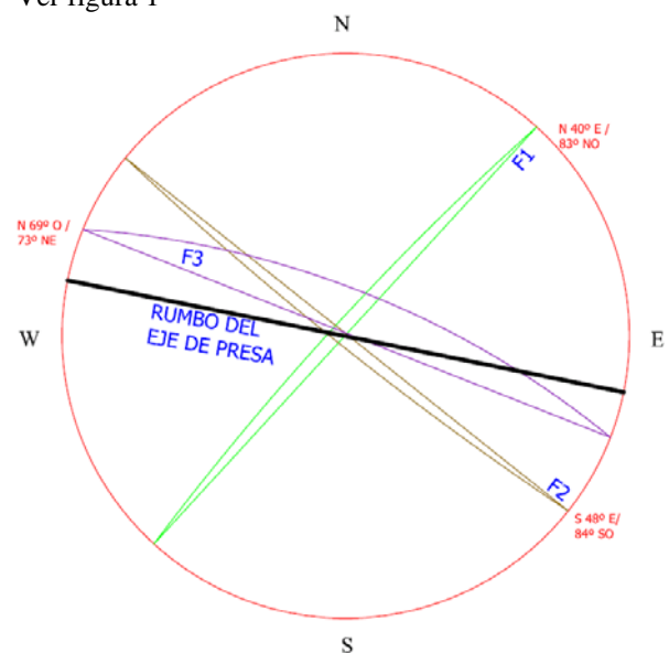
Figura 1. Representación en la red estereográfica de los promedios de las tres familias de fracturas y el eje de Presa.
