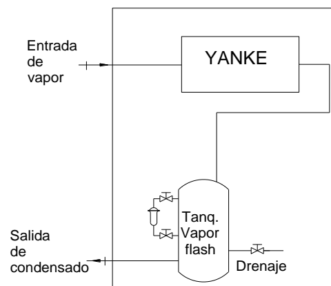
Figura 3.6. Balance de energía en el subsistema 2
