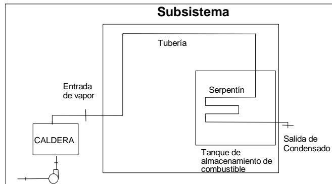
Figura 3.5. Balance de energía en el subsistema 1
