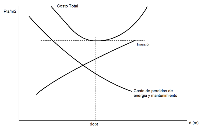
Figura 5.2. Espesor óptimo económico de aislamiento térmico
