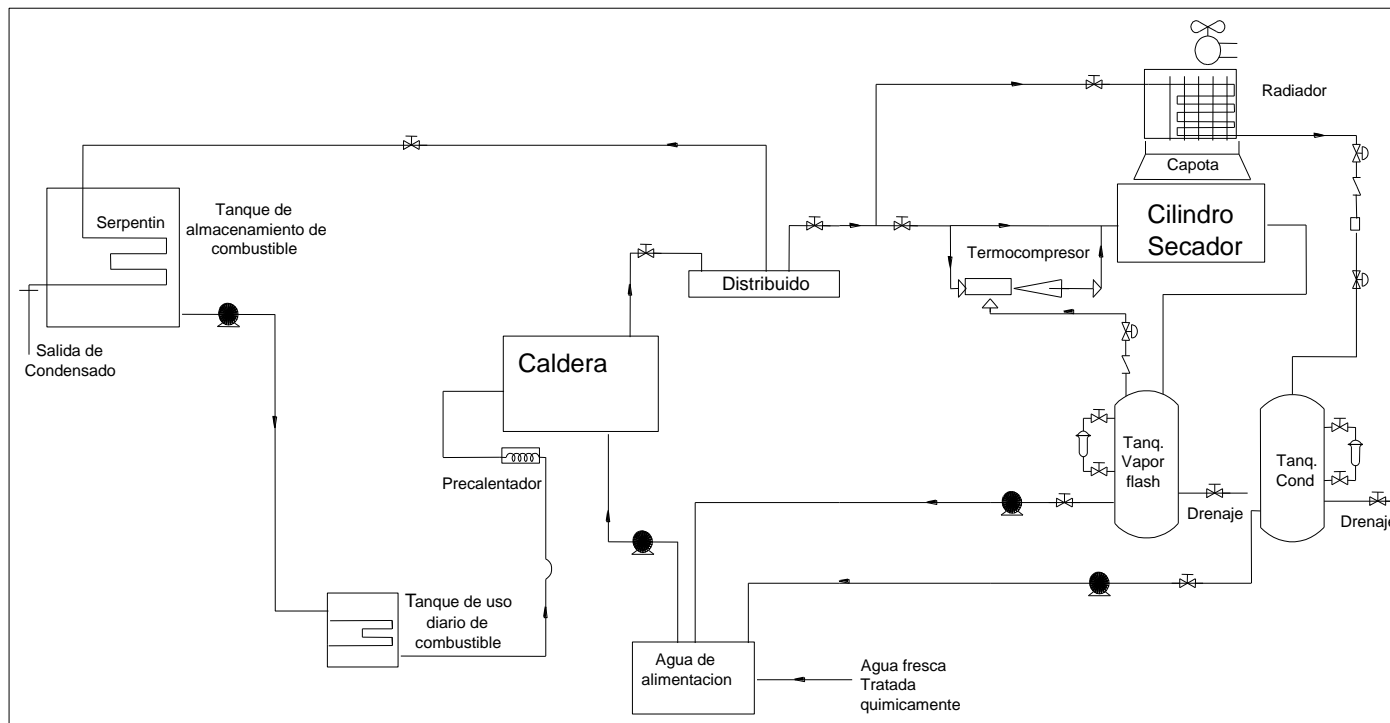
Figura 3.1. Diagrama (PIED) equipos utilizados en el proceso
