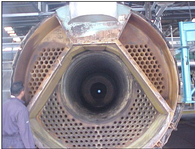
Figura 5.1. Espejo de la caldera
