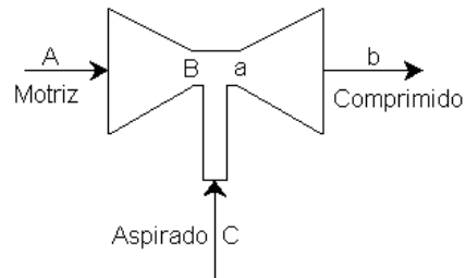
Figura 3.2. Recuperación de vapor en el termocompresor
