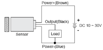
< PNP output >
