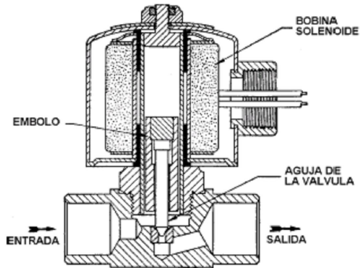
Figura 15: Gráfico de una electroválvula
