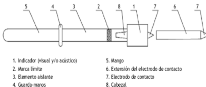
Fig. 5.5a. Detector de tensión tipo capacitivo para AT. (Fuente: Guía Técnica para la Evaluación y Prevención de Riesgo Eléctrico)
