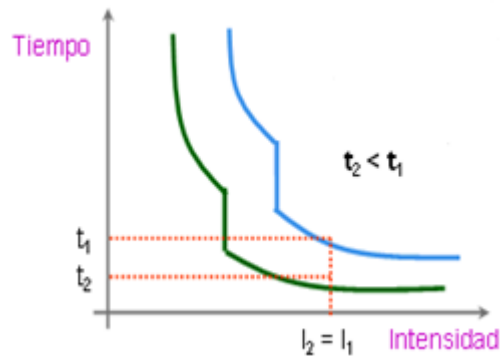
Fig. 3.7. Selectividad Cronométrica. (Fuente: http://www.tuveras.com/aparamenta/magnetotermico.htm )
