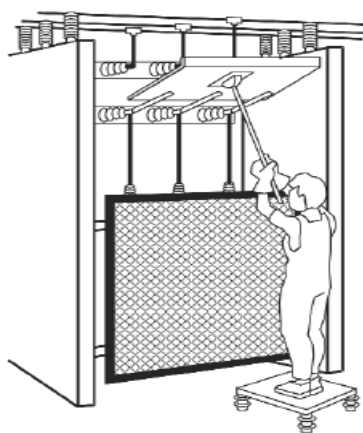
Fig. 5.4. Colocación de láminas aislantes. (Fuente: Guía Técnica para la Evaluación y Prevención de Riesgo Eléctrico)
