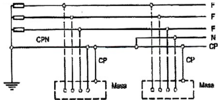
Fig. 2.9. Esquema TN-C-S. (Fuente: http://www.coitiab.es/reglamentos/electricidad/reglamentos/itc_bt/itc-bt-08.htm )
