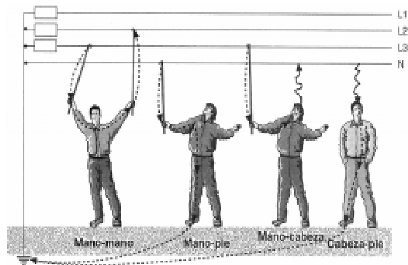
Fig. 1.4. Recorrido de la corriente por el cuerpo humano. (Fuente: Riesgo Eléctrico - Manuel Miguel Delgado Carranza)
