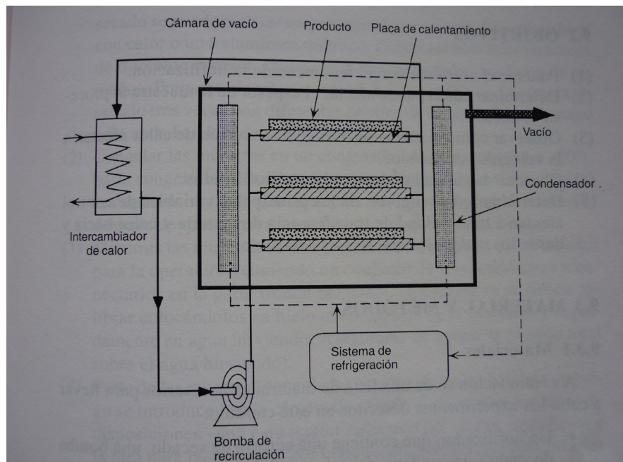
Fig1. 1. Esquema de un sistema Liofilizador
