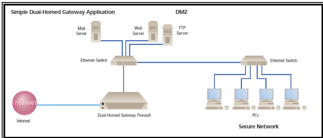
Figura 1.20 Ejemplo de una red con zona desmilitarizada.
