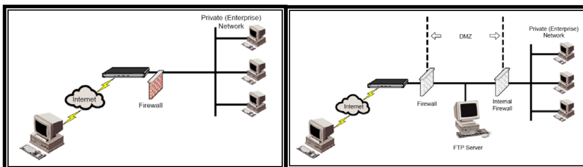
Figura 1.9 Topologías de Redes con Firewall.
