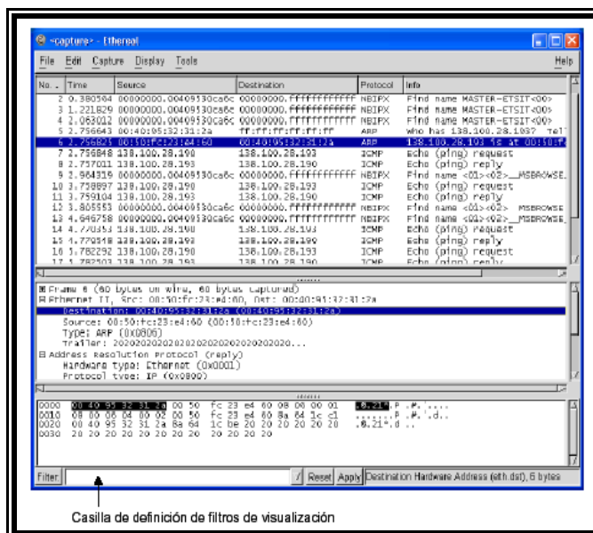
Figura 1.5 Aspecto de la ventana principal del analizador:
