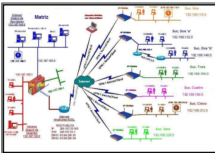
Figura 1.4 Bosquejo de una Estructura de red grande.
