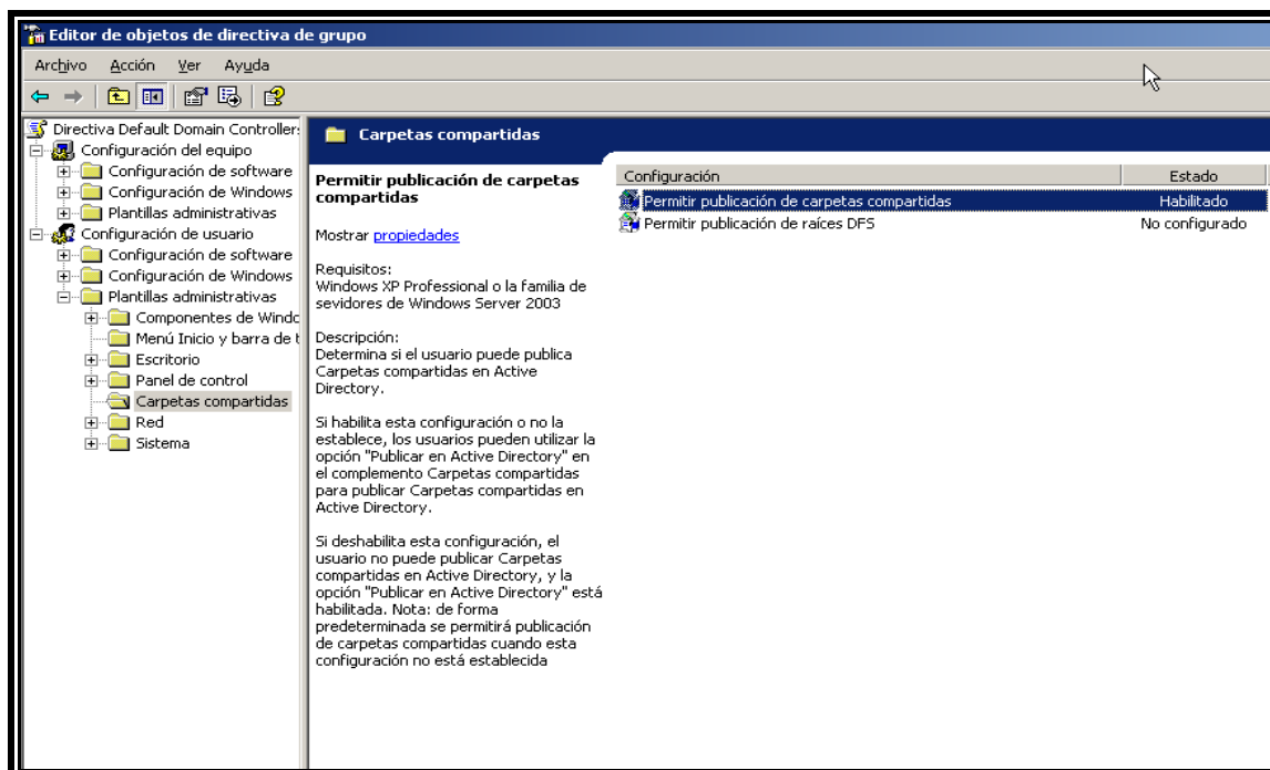
Figura 4.7 Compartición de Carpetas configurada
