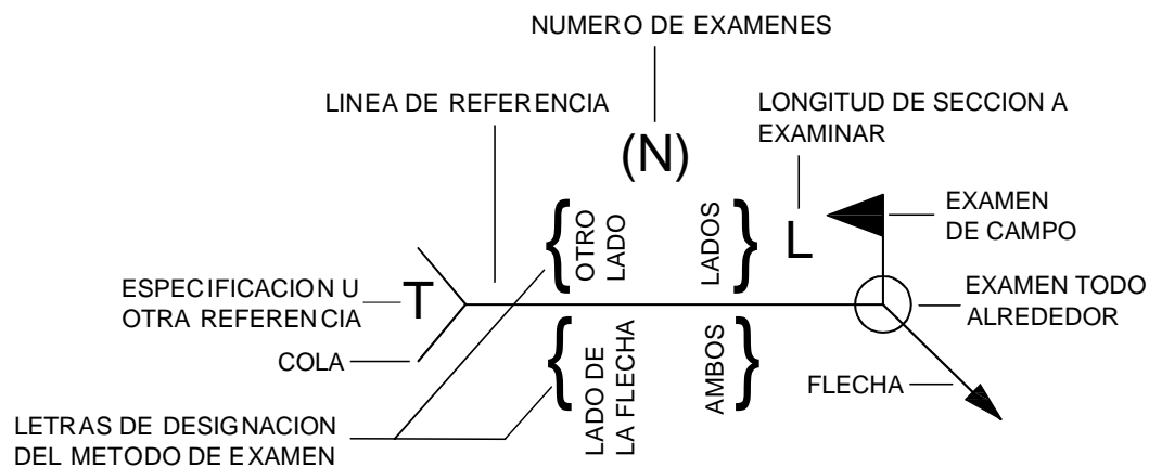
FIGURA 3.4 UBICACIÓN NORMALIZADA DE LOS ELEMENTOS DE END (9)
