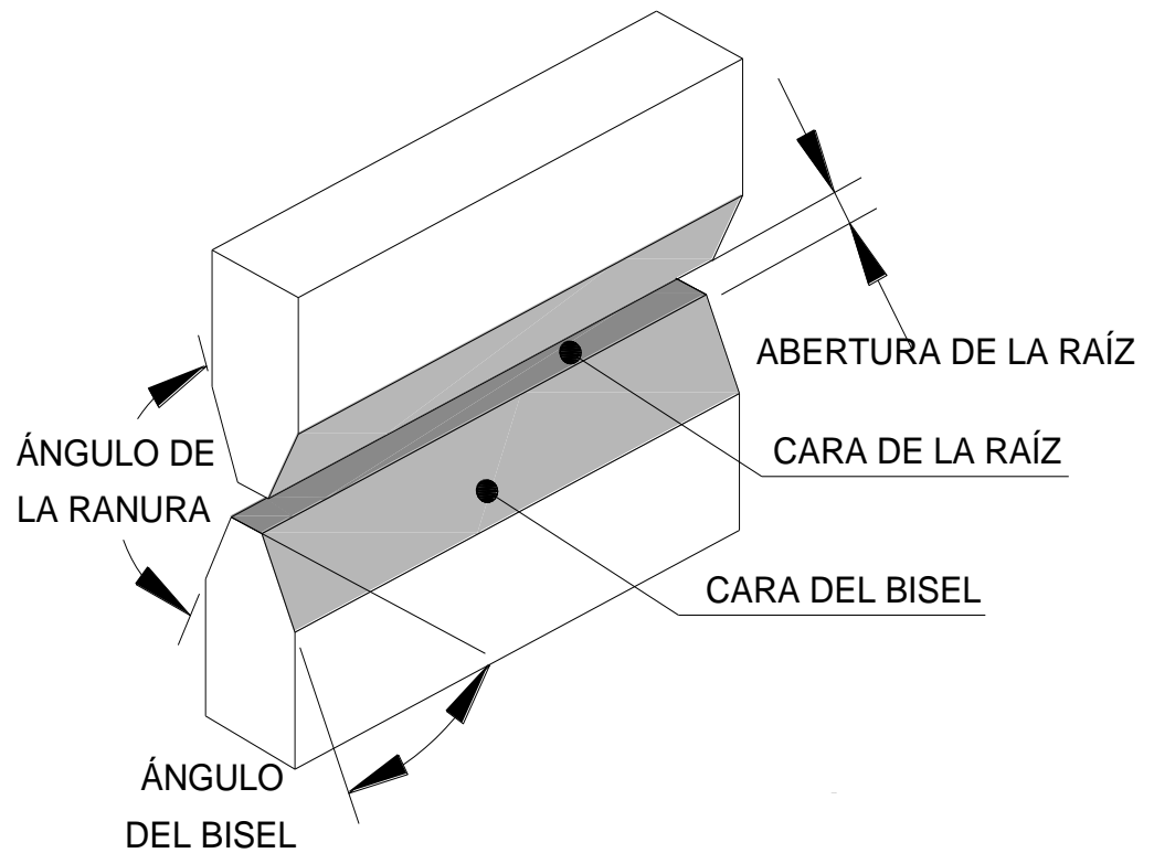
FIGURA 3.7 PARTES DE UNA JUNTA DE RANURA (3)
