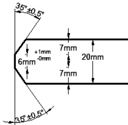
FIGURA 2.2 DIMENSIONES Y TOLERANCIA DE BISEL (1)
