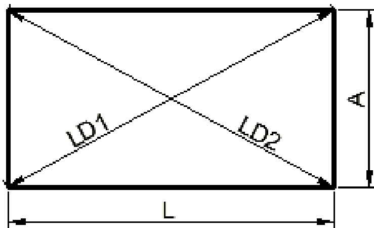
FIGURA 2.1 PARÁMETROS DE CONTROL DIMENSIONAL (6)
