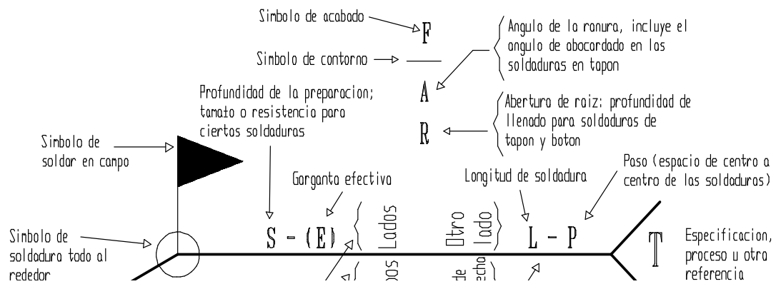
FIGURA 3.2 SITUACIÓN NORMALIZADA DE LOS ELEMENTOS DE UN SÍMBOLO DE SOLDADURA (3)
