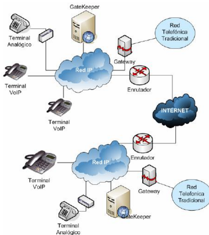
Figura2.1 Estructura Básica de dos delegaciones de una misma empresa conectadas telefónicamente a través de Internet
