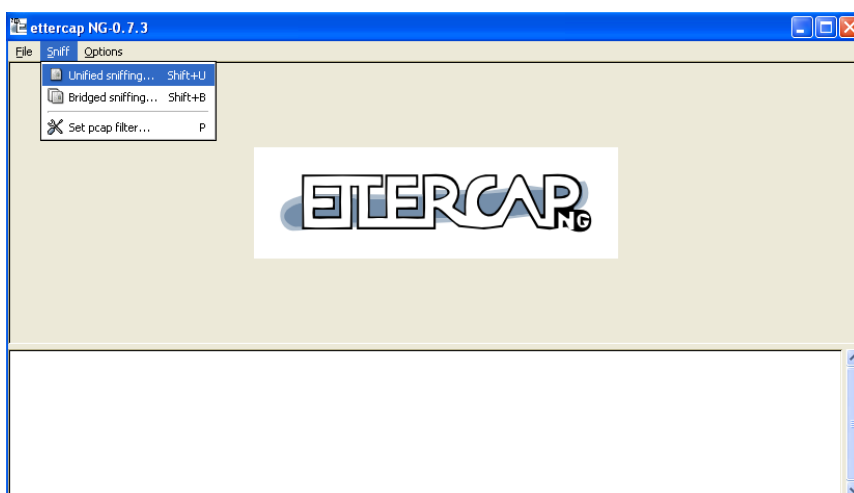
Figura 3.9 Paso1 Ettercap
