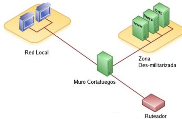
Figura 4.2 Grafica de las 3 interfaces del Cortafuego Shorewall
