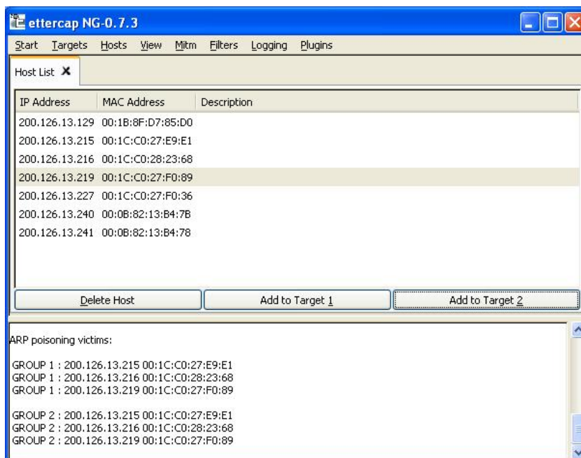
Figura 3.13 MitM con Ettercap
