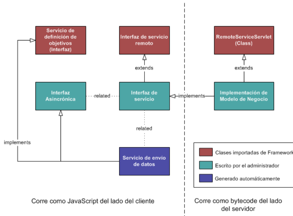
Figura 7. Estructura de aplicación web usando GWT. [7]
