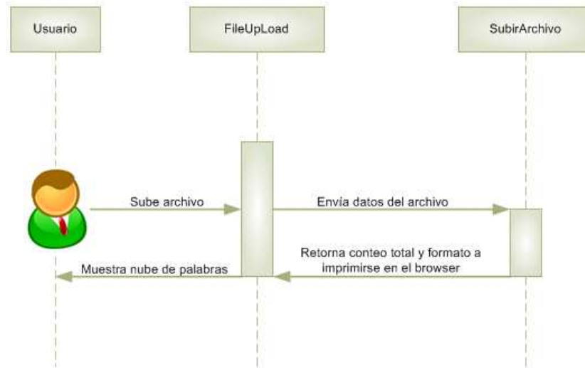
Figura 6. Diagrama Interacción Objeto Escenario 4.1
