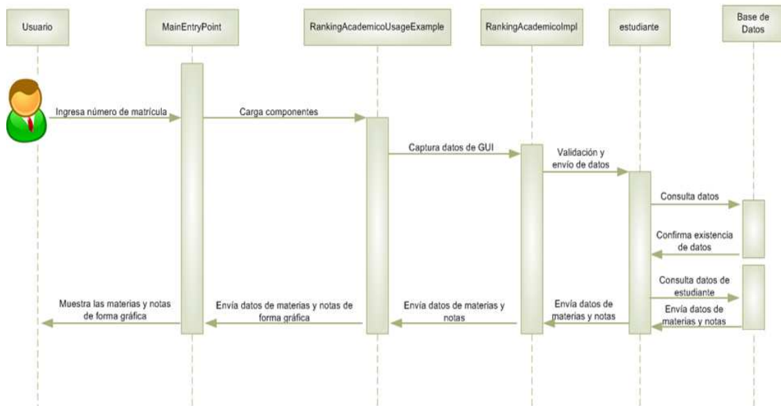
Figura 5. Diagrama Interacción Objeto Escenario 3.1
