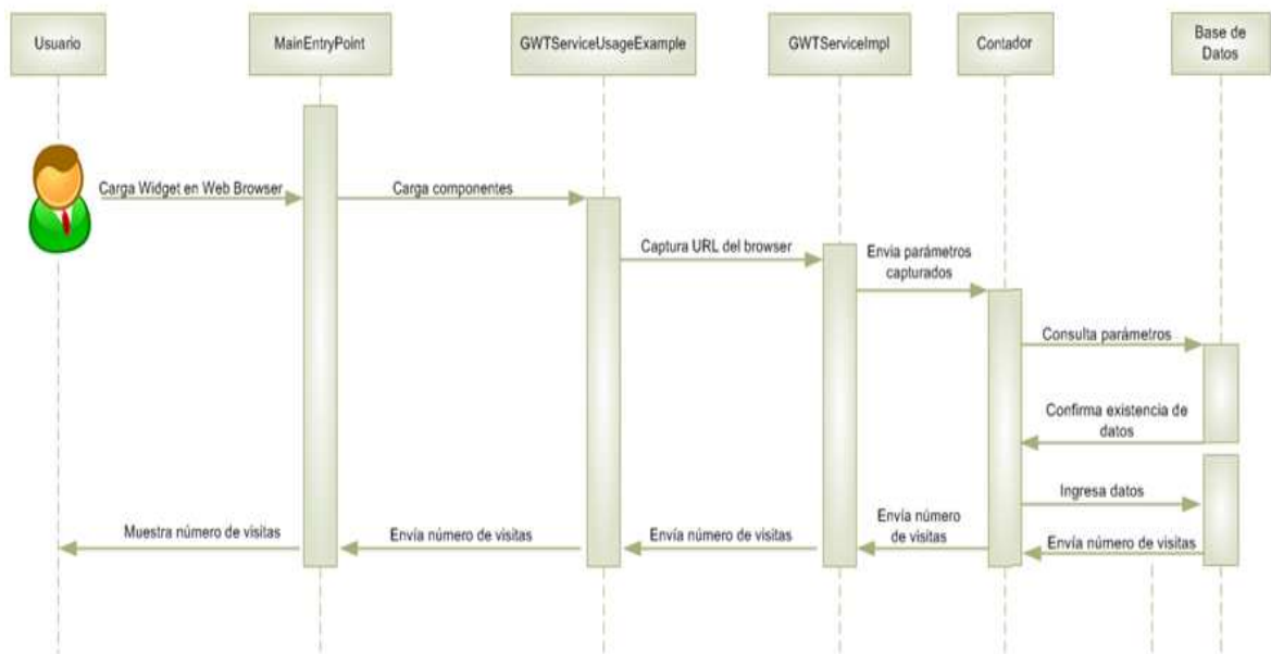
Figura 4. Diagrama Interacción Objeto Escenario 2.1
