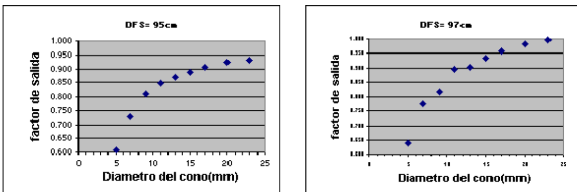
Fig. 3.6 Variación del factor de salida respecto al diámetro del colimador circular, normalizada la salida al campo de 10 \times 10 \text{cm}^2
