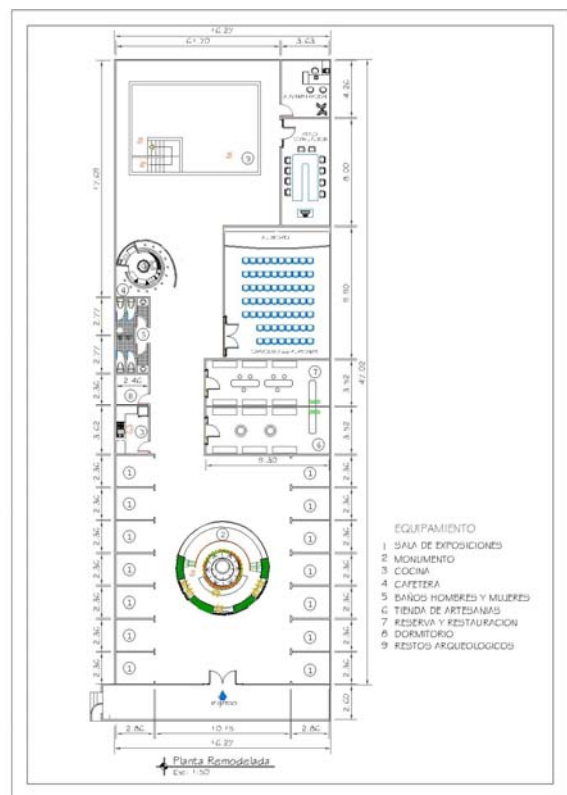
Figura 2. Plano del proyecto propuesto
