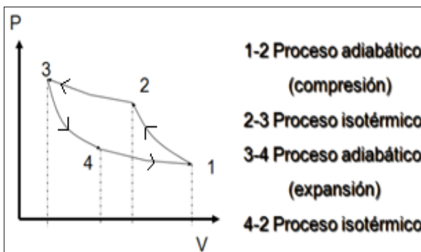
FIG-2.8 CICLO DE CARNOT PARA MAQUINA FRIGORÍFICA
