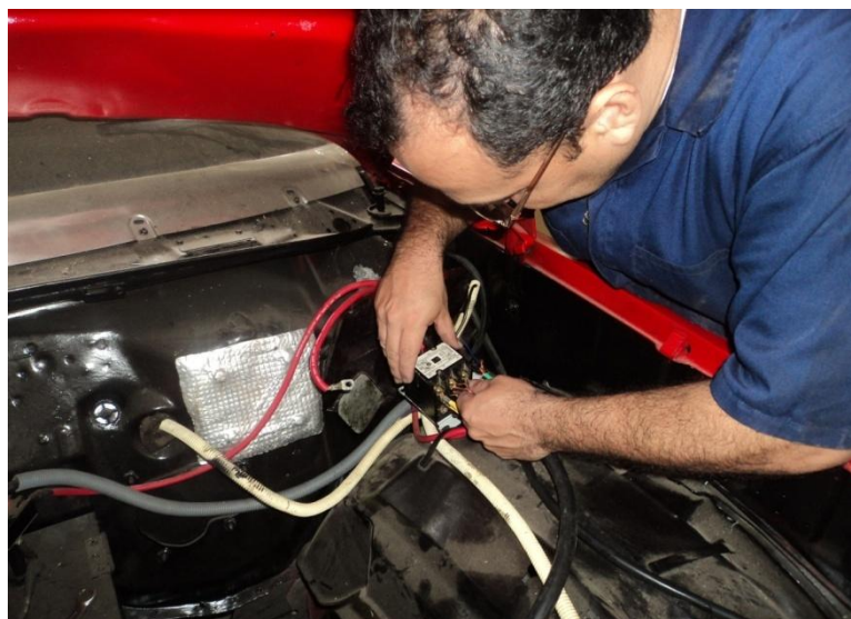
FIG-4.36 REVISIÓN DEL CONTACTOR
