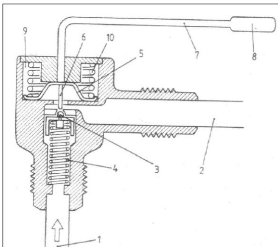
FIG-2.23 ESQUEMA DE LA VÁLVULA DE EXPANSIÓN.
