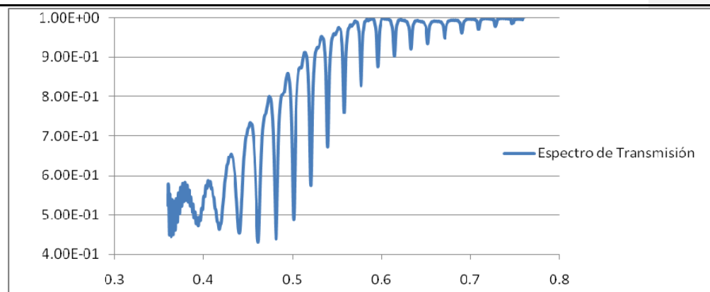
Figura 11: Gráfico Frecuencia vs Espectro(Paso)
