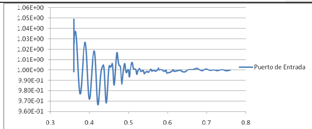
Figura 10: Gráfico Frecuencia vs Espectro(Entrada)
