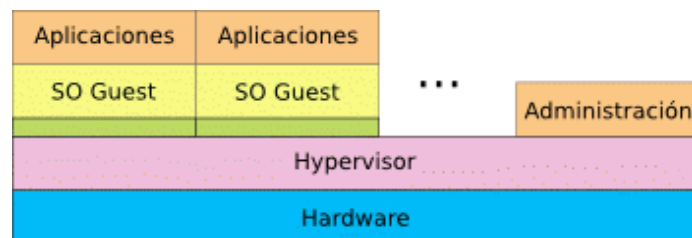
Fig. 2.4 Paravirtualización
