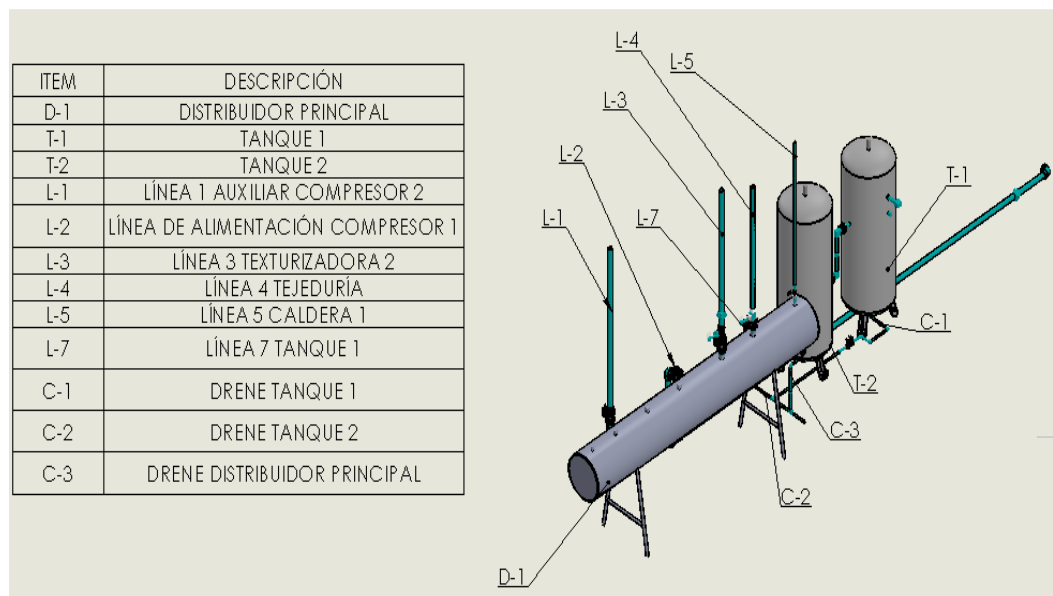
FIG. 2.13 DISTRIBUIDOR PRINCIPAL
