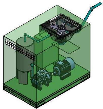
VISTA DE DETALLE A COMPRESOR 2 POTENCIA: 112KW PRESIÓN: 12 BAR CAPACIDAD: 16MCM
