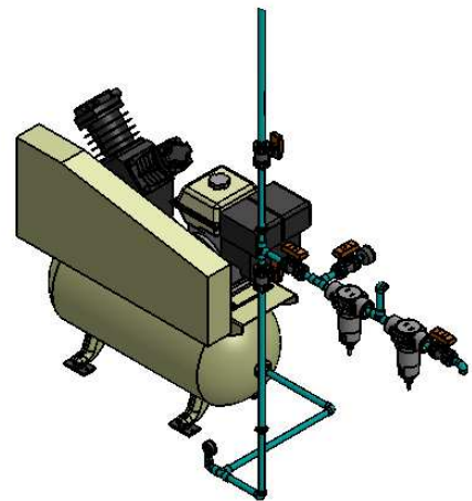
VISTA DE DETALLE D COMPRESOR 3 POTENCIA: 3.73KW PRESIÓN: 10 BAR CAPACIDAD: 0.57MCM
