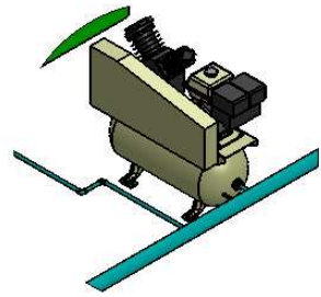
VISTA DE DETALLE F COMPRESOR 4 POTENCIA: 0.75KW PRESIÓN: 10 BAR CAPACIDAD: 0.18 MCM
