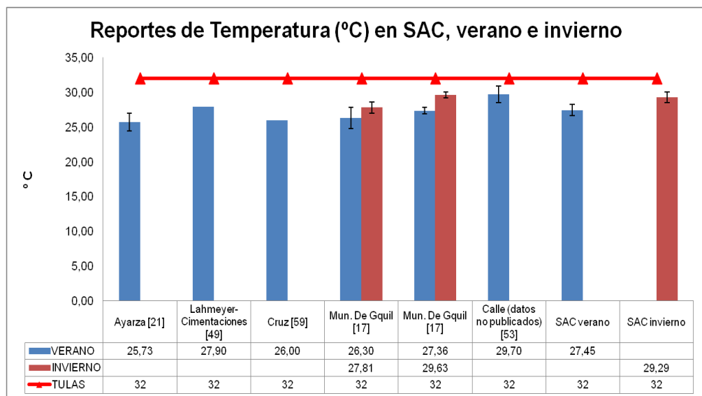
Figura 40 a. Reportes de temperatura de años anteriores en SAC
