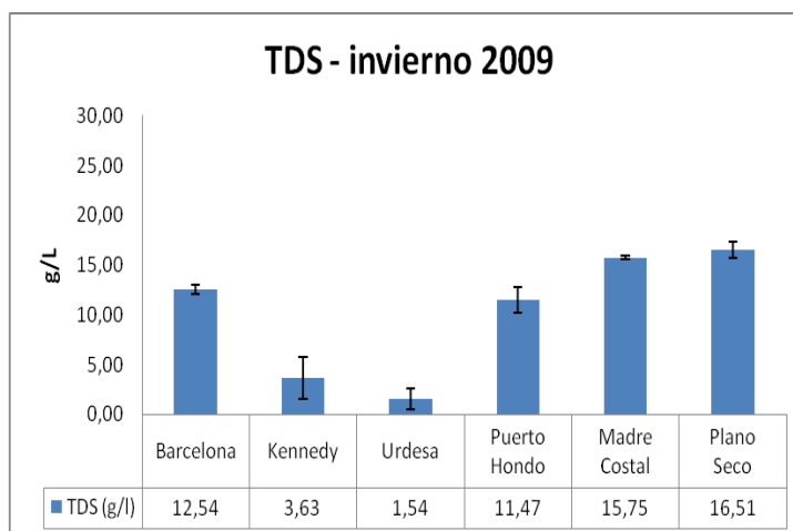
Figura 27 a. Valores promedios de TDS encontrados en cada estación de estudio, invierno 2009
