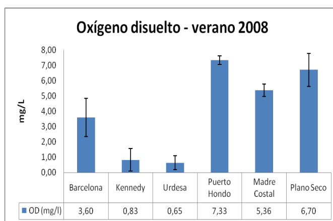
Figura 11a. Valores promedios de oxígeno disuelto en cada estación de estudio, verano 2008
