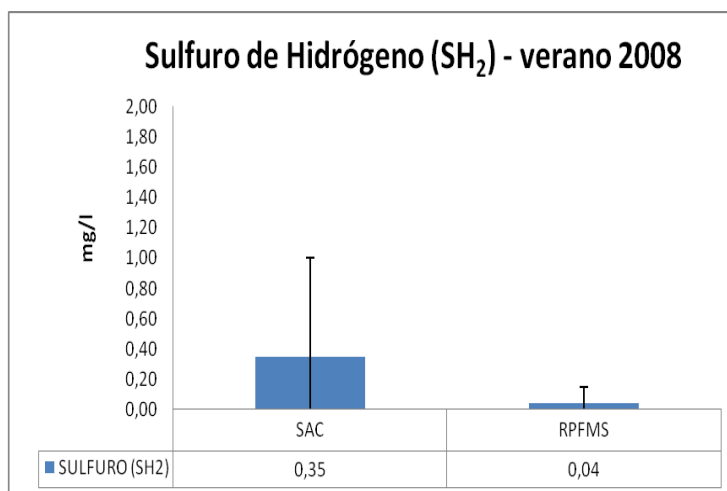
Figura 16 b. Valores promedio de SH 2 en SAC y en el sector de la RPFMS, verano 2008
