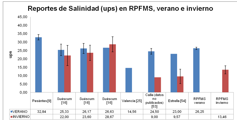
Figura 42 b. Reportes de salinidad de años anteriores en RPFMS
