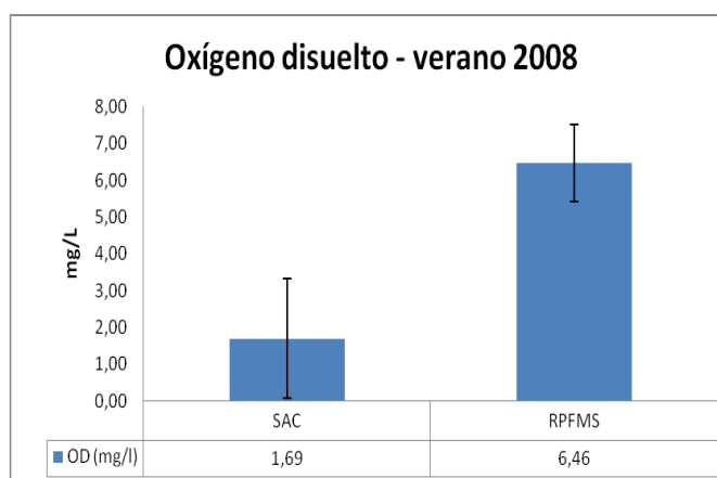
Figura 11b. Valores promedios de oxígeno disuelto en SAC y en el sector de la RPFMS, verano 2008
