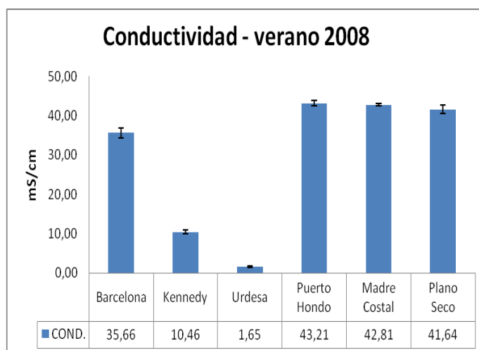
Figura 15 a. Valores promedios de conductividad en cada estación de estudio, verano 2008
