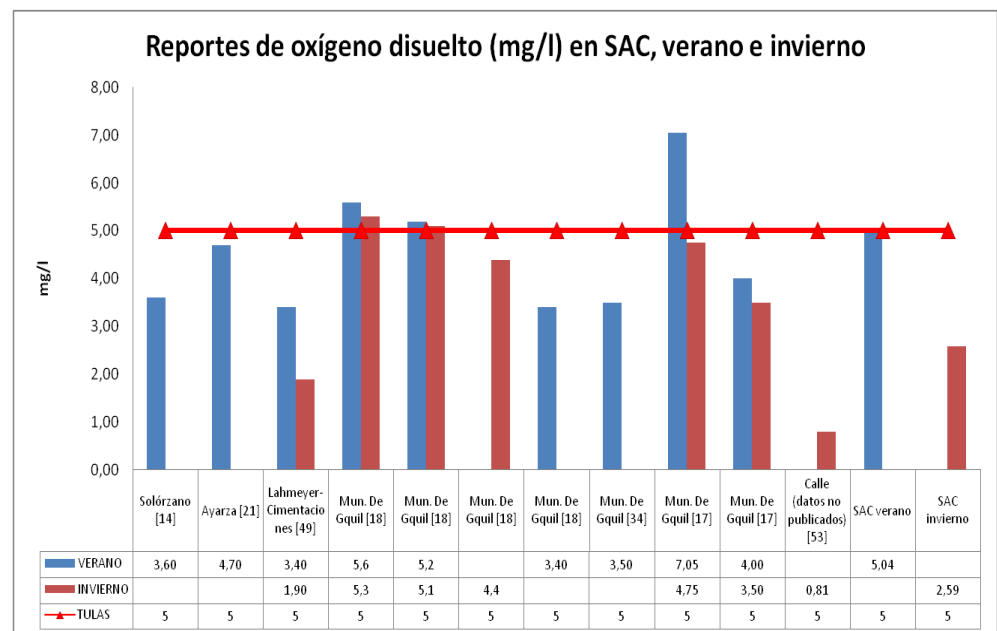
Figura 41 a. Reportes de oxígeno disuelto de años anteriores en SAC.
