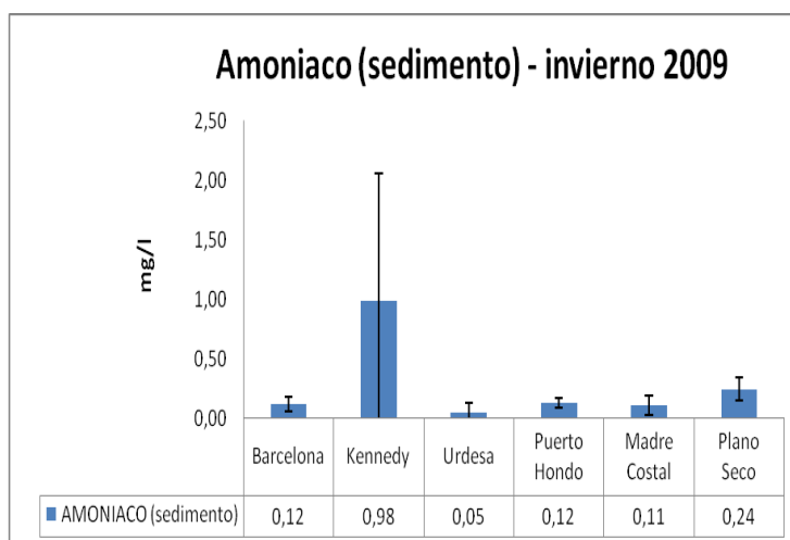
Figura 35 a. Valores promedios de amoniaco en sedimento en cada estación de estudio, invierno 2009
