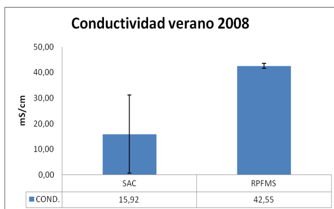
Figura 15 b. Valores promedios de conductividad en SAC y en el sector de la RPFMS, verano 2008
