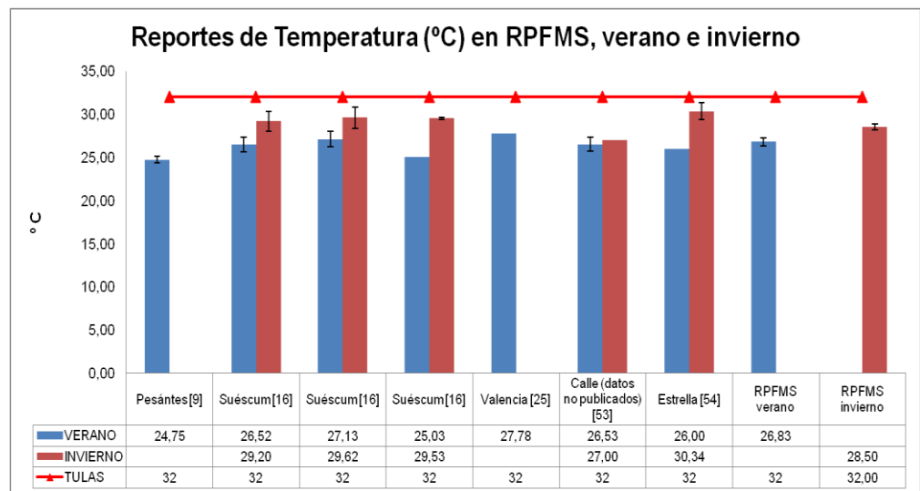
Figura 40 b. Reportes de temperatura de años anteriores en RPFMS
