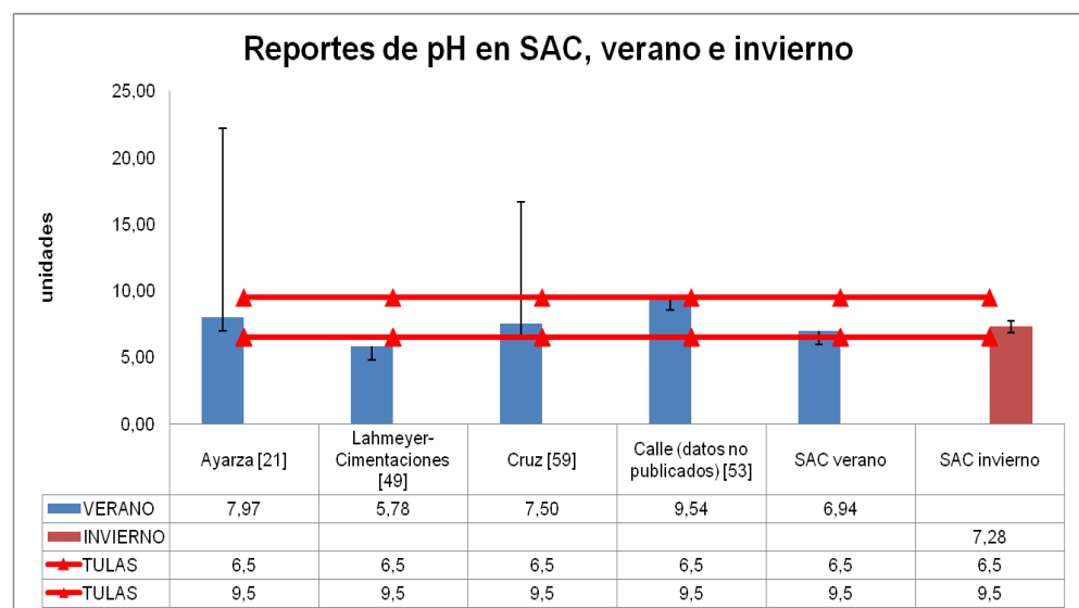
Figura 43 a. Reportes de pH de años anteriores en SAC
