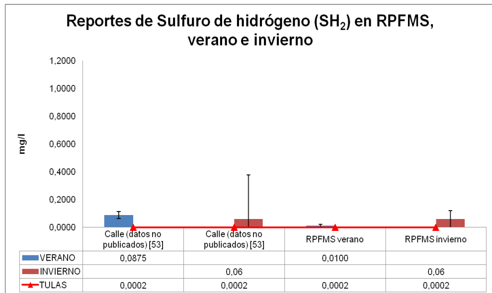
Figura 44 b. Reportes de sulfuro de hidrógeno de años anteriores en RPFMS
