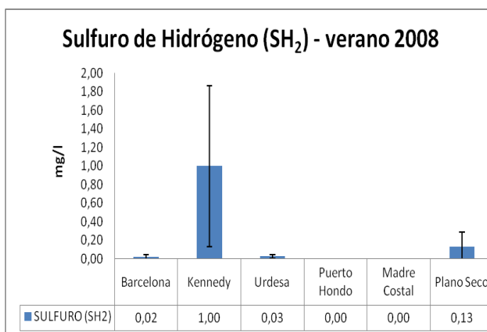
Figura 16 a. Valores promedios de SH 2 en cada estación de estudio, verano 2008
