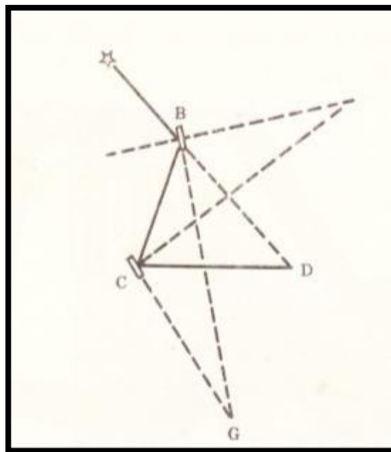
Figura 2-5 Principio Óptico del Sextante. xxv
