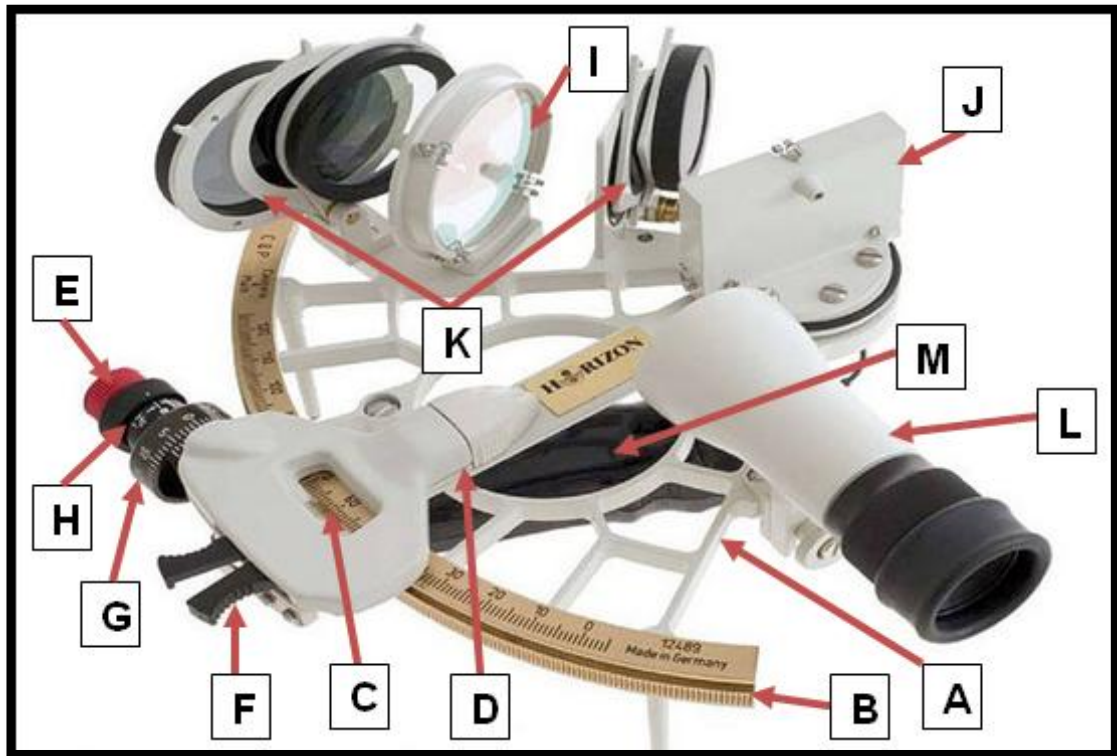
Figura 2-1 Descripción del Sextante. xxi
