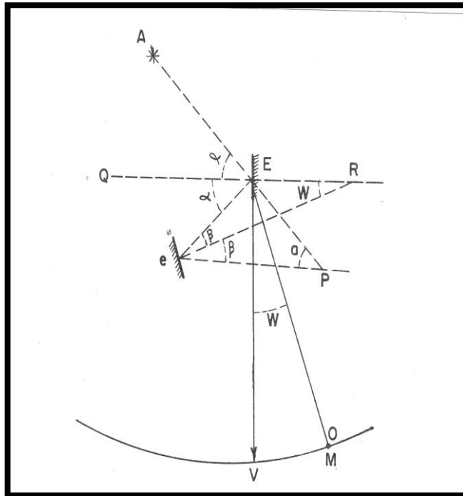
Figura 2-4 Teorías del Sextante está Basada en las dos Leyes de la Reflexión de la Luz. xxiv
