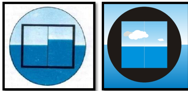
Figura 3-6 Espejo Índice con El Espejo del Horizonte. xxxiii
