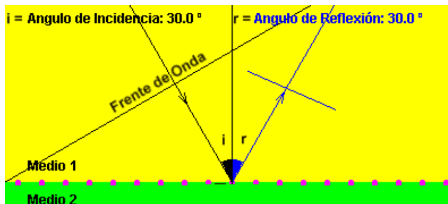
Figura 2-7 Ángulos Iguales en el Plano. xxvii
