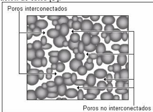
Figura 1. Representación de la porosidad en una roca reservorio.
