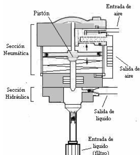
Figura 4. Esquema interno de la bomba hidráulica
