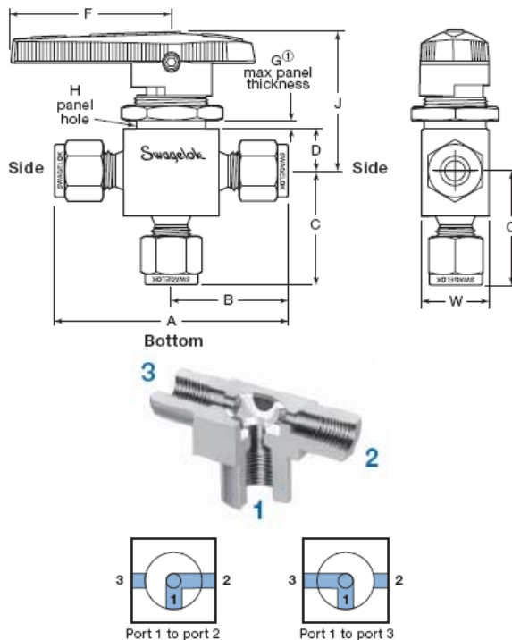
Figura 7. Válvula de tres vías y posiciones de flujo
