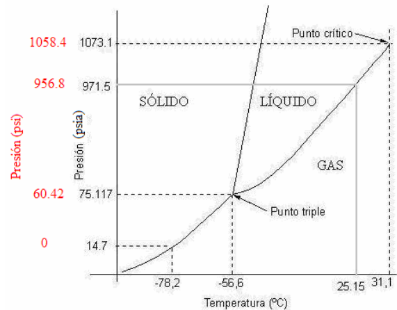
Figura 2. Diagrama de fases del CO 2 .
