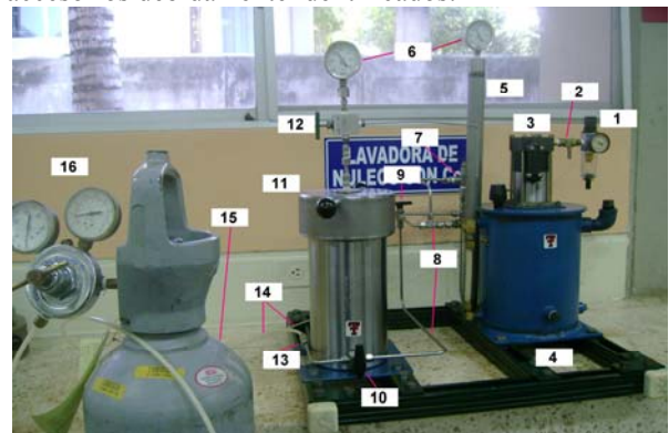
Figura 3. Partes que conforman el limpiador de núcleos con CO 2 .
