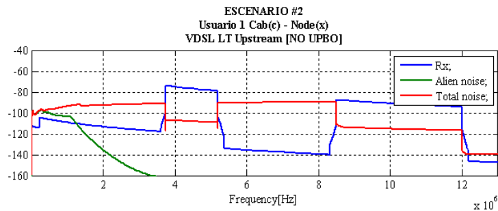
Figura 3.15 Simulación del Escenario 2, Usuario 1, sin UPBO
