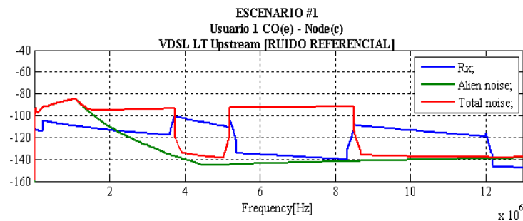
Figura 3.13 Simulación del Escenario 1, Usuario 1, con Ruido Referencial
