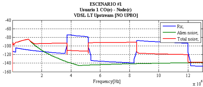
Figura 3.5 Simulación del Escenario 1, Usuario 1, sin UPBO
