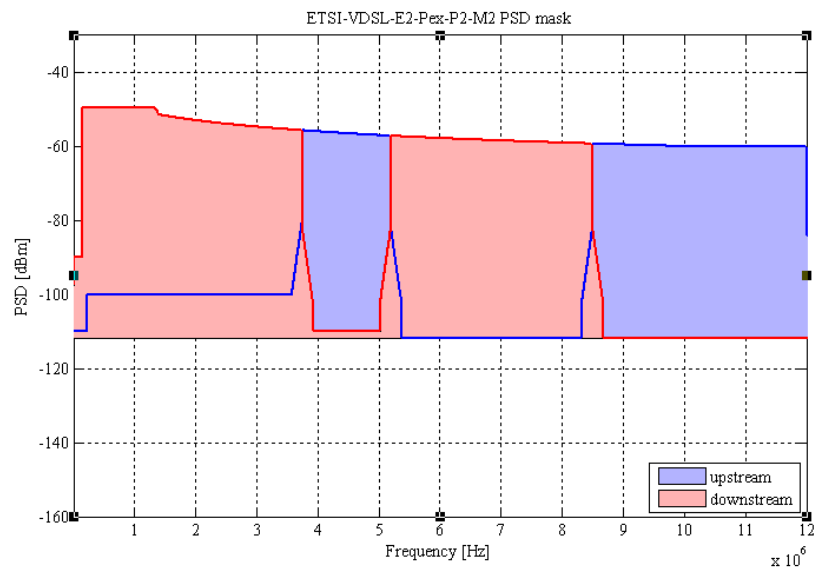
Figura 3.2 Máscara E2-Pex-P2-M2 utilizada para el Escenario 1
