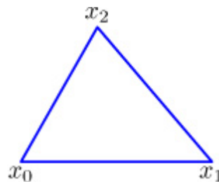
Figura 2.1 Triángulo de análisis definido por Nelder-Mead para \Phi
