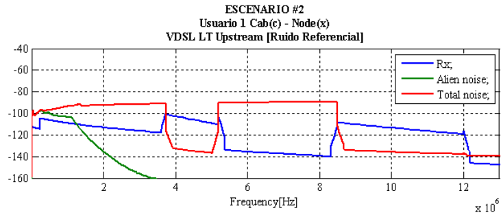
Figura 3.23 Simulación del Escenario 2, Usuario 1, con Ruido Referencial
