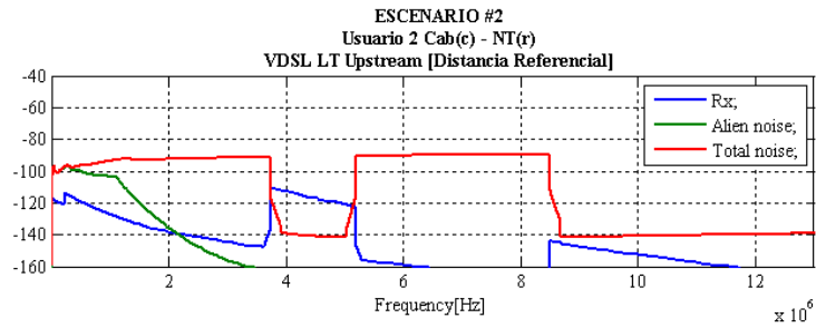
Figura 3.20 Simulación del Escenario 2, Usuario 2, con Distancia Referencial
