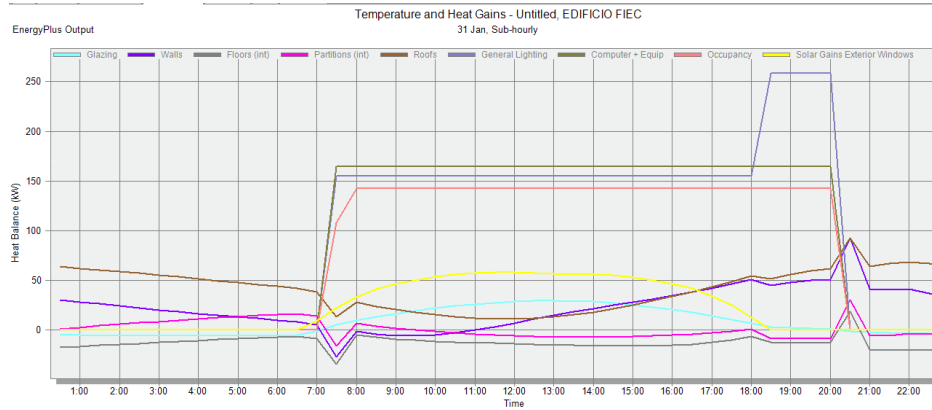
Figura A-7. Ganancias Caloríficas Modelo 5.
