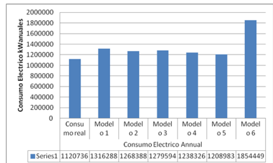
FIGURA 12. COMPARACIÓN DE GASTO ELÉCTRICO.
