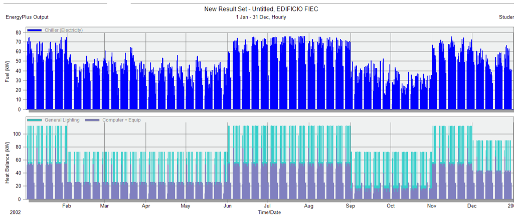
Figura A-4. Consumo Energético Modelo 3.
