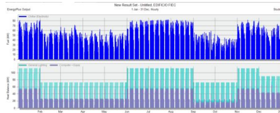
Figura 5. Consumo Energético Modelo 1.
