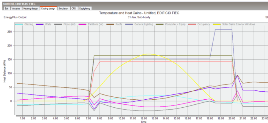
Figura A-3. Ganancias Caloríficas Modelo 3.
