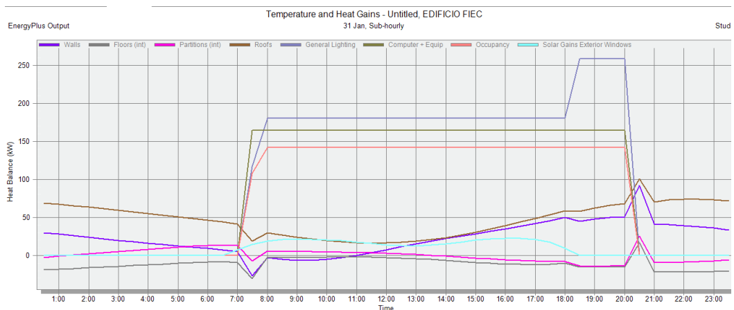
Figura A-9. Ganancias Caloríficas Modelo 6.
