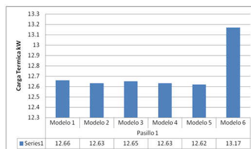
FIGURA 8. COMPARACIÓN DE CARGAS TÉRMICAS DEL PASILLO 1
