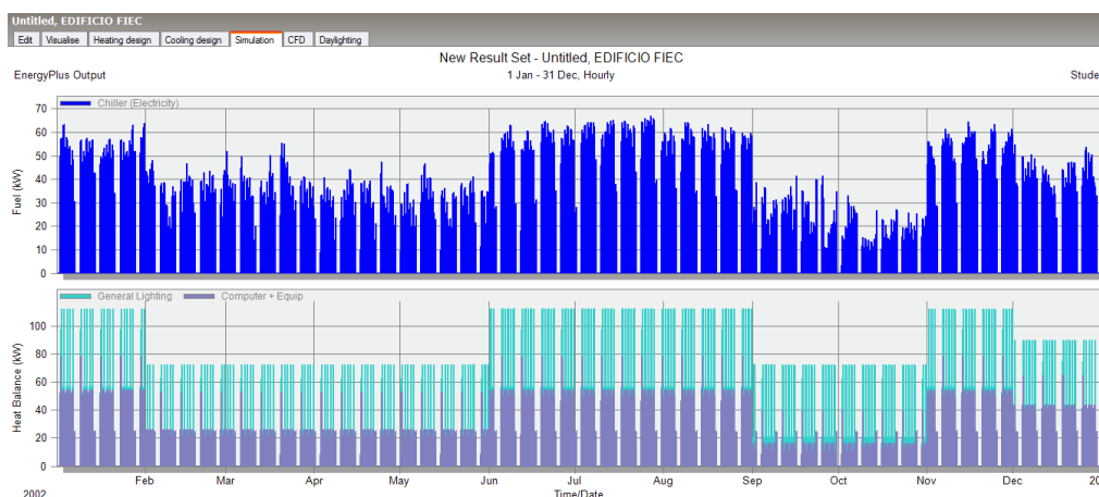
Figura A-6. Consumo Energético Modelo 4.
