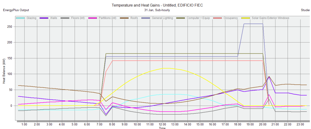
Figura A-1. Ganancias Caloríficas Modelo 2.
