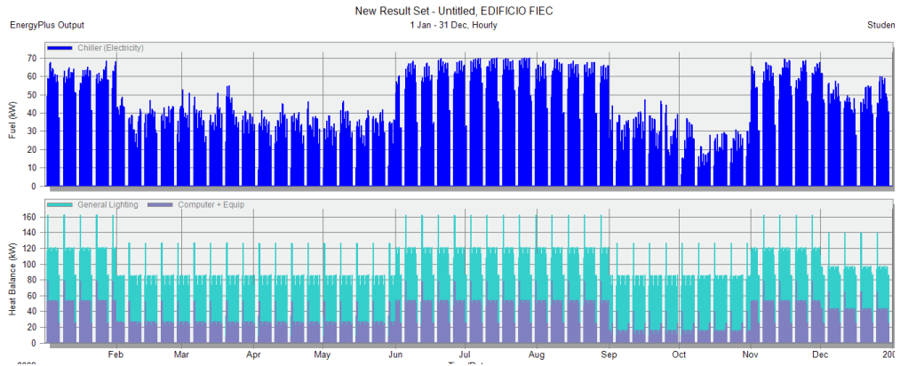
Figura A-10. Consumo Energético Modelo 6.
