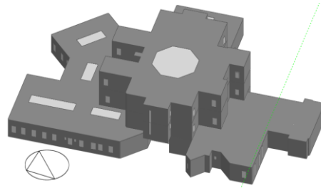
Figura 1. Vista del Edificio de la Facultad de Ingeniería Eléctrica y comunicación en el programa Design Builder.
