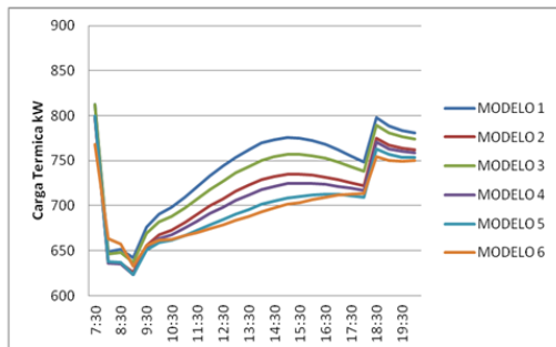
FIGURA 10. COMPARACIÓN DE CARGA TÉRMICA DE CADA MODELO
