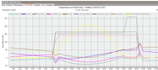
Figura 4. Ganancias de Calor Modelo 1.
