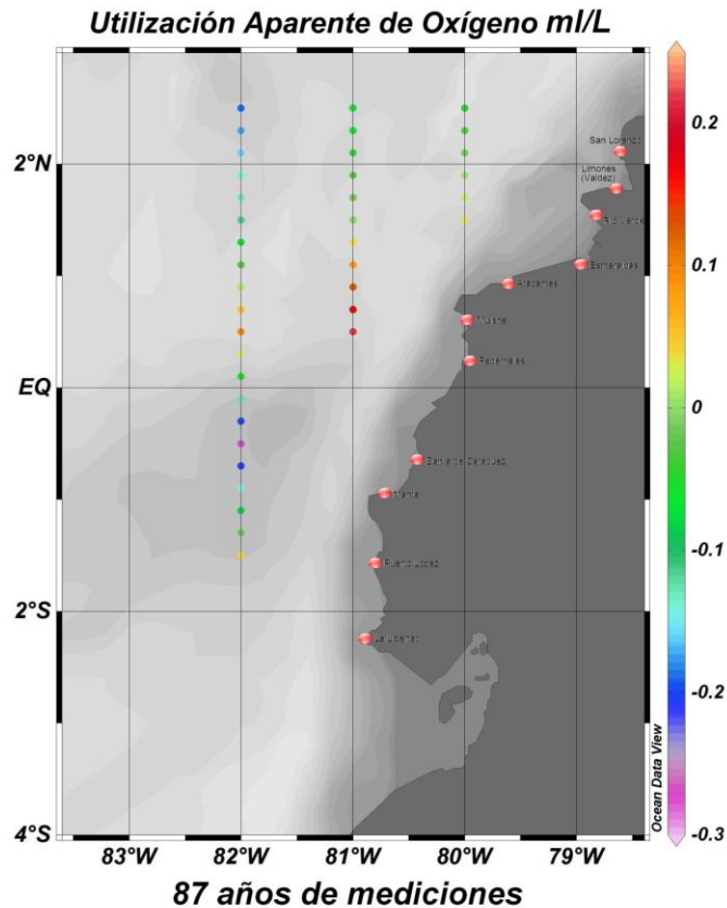
FIGURA 3.2.- Fluctuaciones de (UAO) frente a las costas de Ecuador Fuente: García A. Ocean Data View 4
