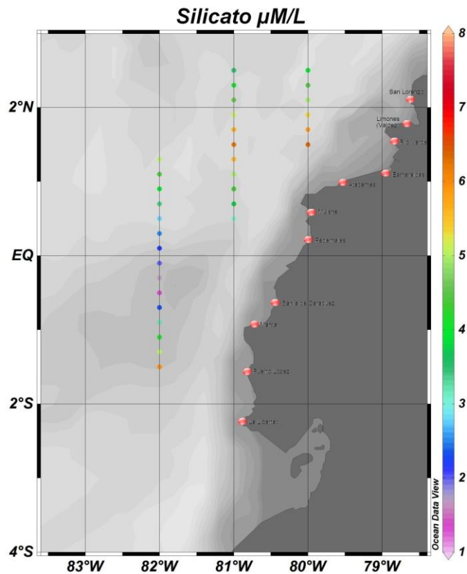
FIGURA 3.4.- Fluctuaciones del Silicato frente a las costas del Ecuador Fuente: García A. Ocean Data View 4
