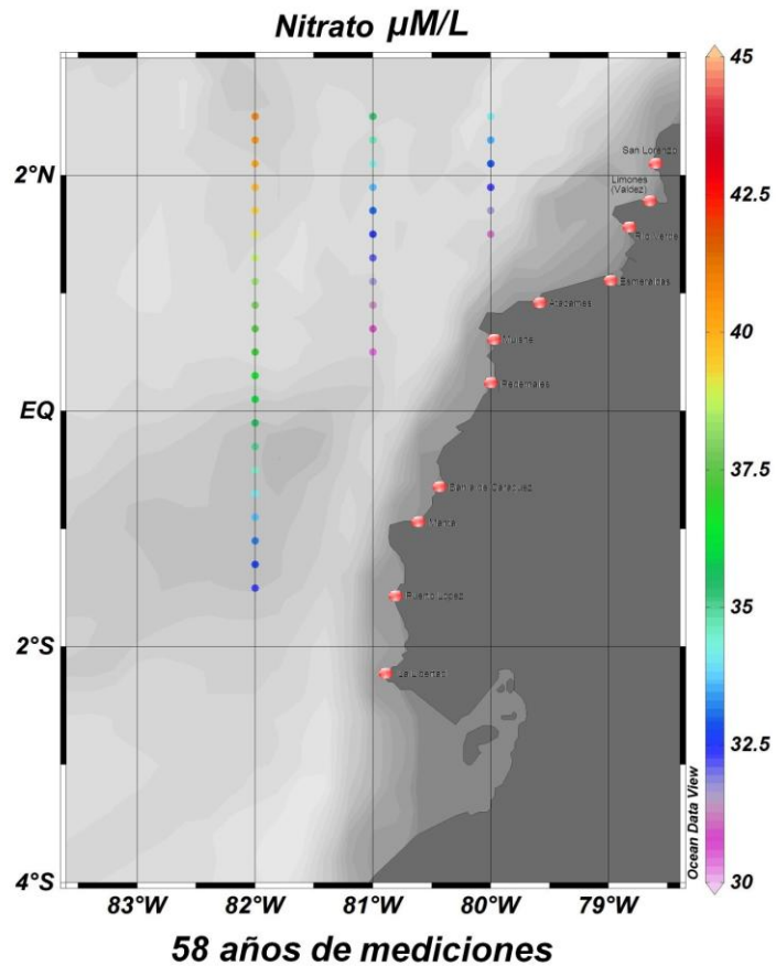
FIGURA 3.8.- Fluctuaciones del Nitrato frente a las costas del Ecuador Fuente: García A. Ocean Data View 4
