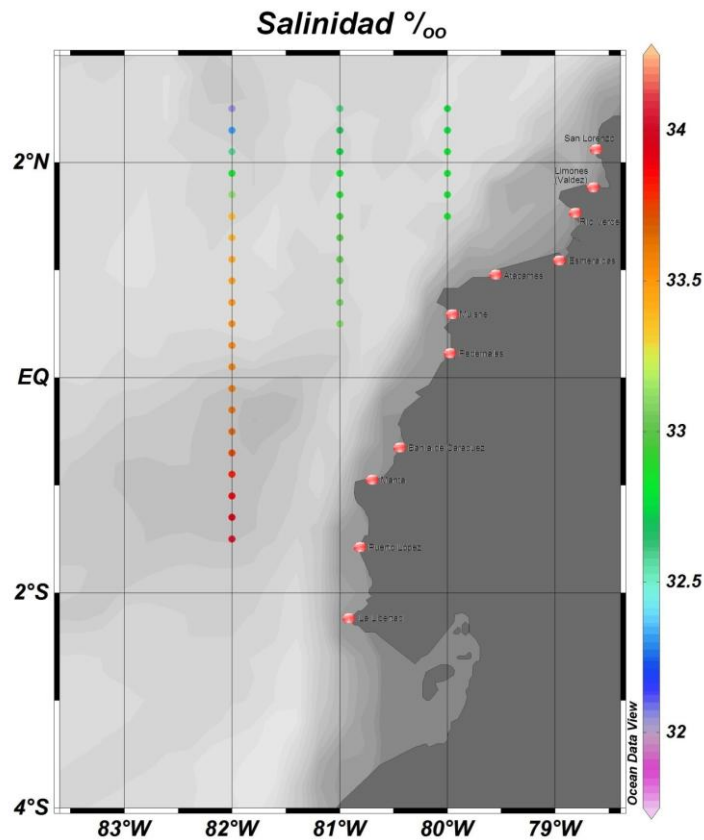
FIGURA 3.5.- Fluctuaciones de la Salinidad frente a las costas del Ecuador Fuente: García A. Ocean Data View 4
