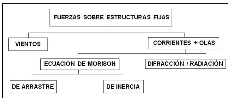
FIGURA 1.13.- TIPO DE FUERZAS SOBRE ESTRUCTURAS FIJAS FONDEADAS EN FUNCIÓN A SU ORIGEN. Fuente:GettyImages
