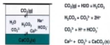
Fig. 1 Algunas reacciones que se generan.
