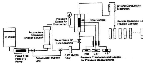
Fig. 3 Equipo normalizado API para ensayos en “cores”
