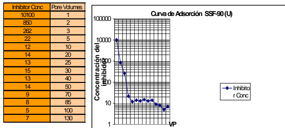
Curva de adsorción para SSF-90 arena U
