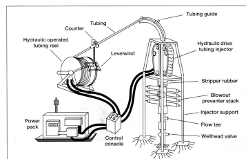
Fig. 2 Unidad de “coiled tubing” y sus componentes
