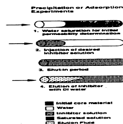
Fig. 4 Procedimiento de inundación del “coreplug”
