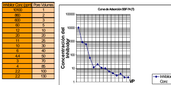
Curva de Adsorción para SSF-74 arena T
