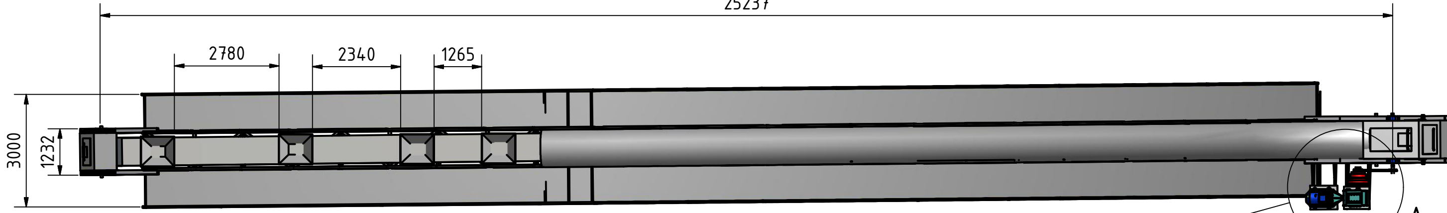
A ( 1 : 50 )Motor, acople y reductor
