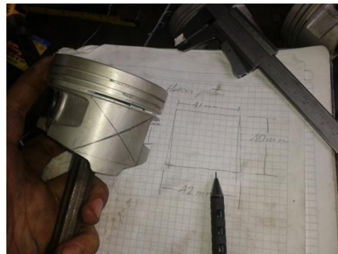
Figura 4-7: Pistón para Mecanizar.
