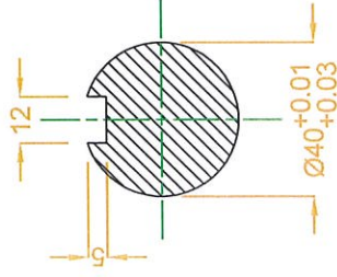
CORTE A-A ESC 1:1
