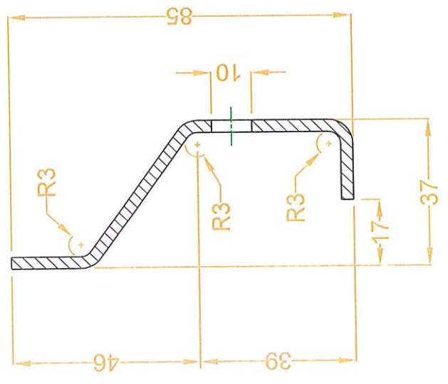
CORTE A-A ESC 1:3
