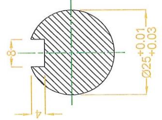
CORTE B-B ESC 1:2
