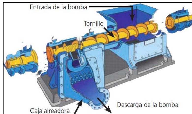
FIGURA 2.6 TRANSPORTE NEUMÁTICO DE TORNILLO (FLS width )
