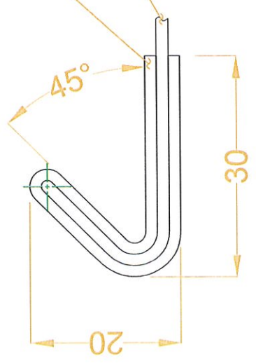
DETALLE 1 ESC 1:10
