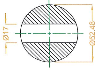
CORTE B-B ESC 1:1
