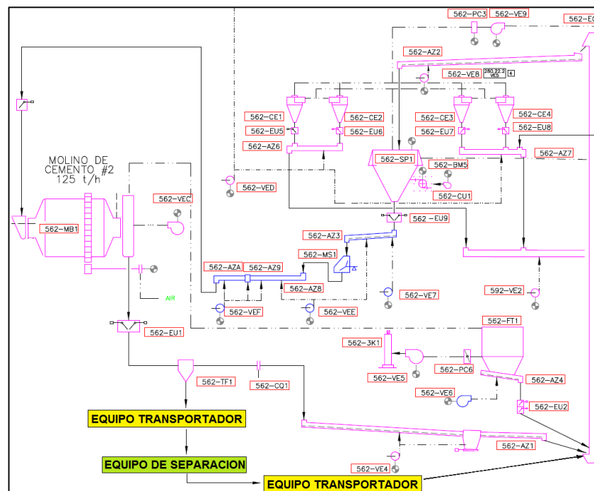
FIGURA 2.9 DIAGRAMA DE FLUJO CEMENTO (Holcim Ecuador S.A.)
