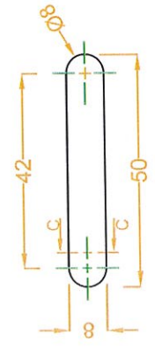
CUÑAS ESC 1:1.5
