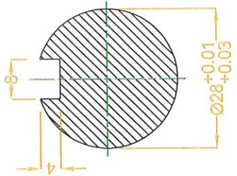
CORTE A-A ESC 1:2
