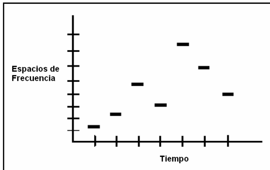
Figura 1.12 Esquema de modulación FHSS
