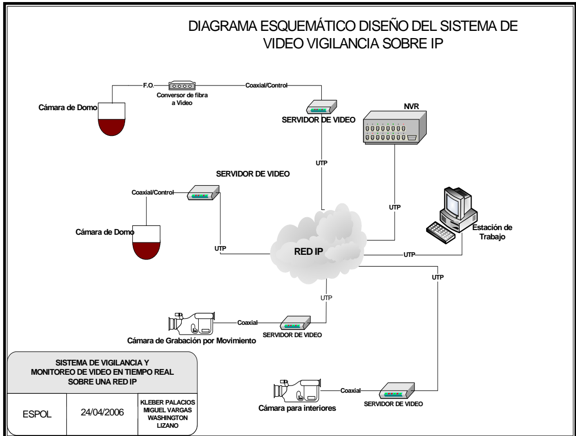
Figura 3.2 Diseño General del Sistema de Video Vigilancia sobre IP
