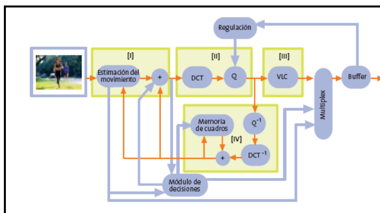
Figura 1.18 Esquema básico de un codificador híbrido.
