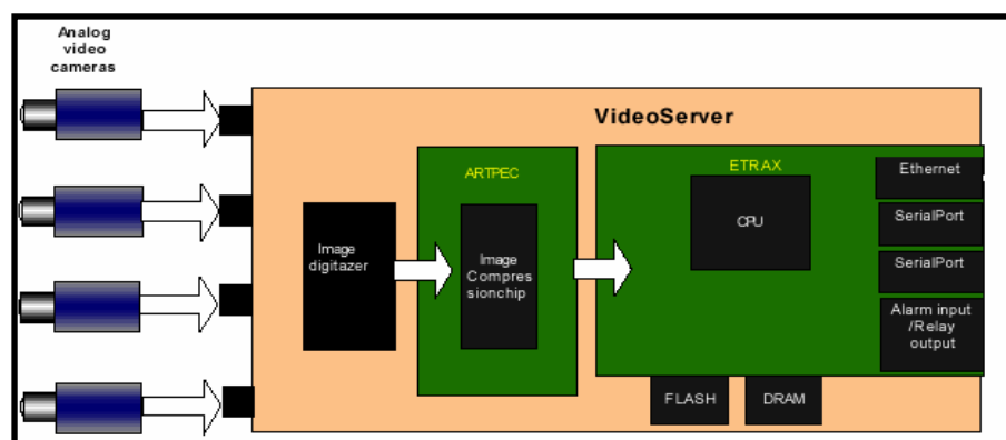
Figura 2.15 Esquema de un servidor de vídeo
