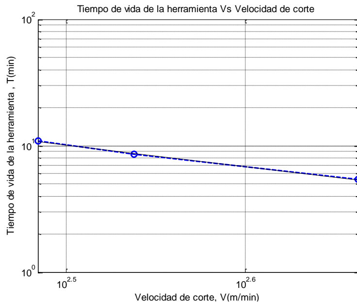
GRÁFICA 3.6 CURVA V-T PARA V_{B_0}=0.3\text{mm} ( V_c=305\text{-}460\text{ m/min} )
