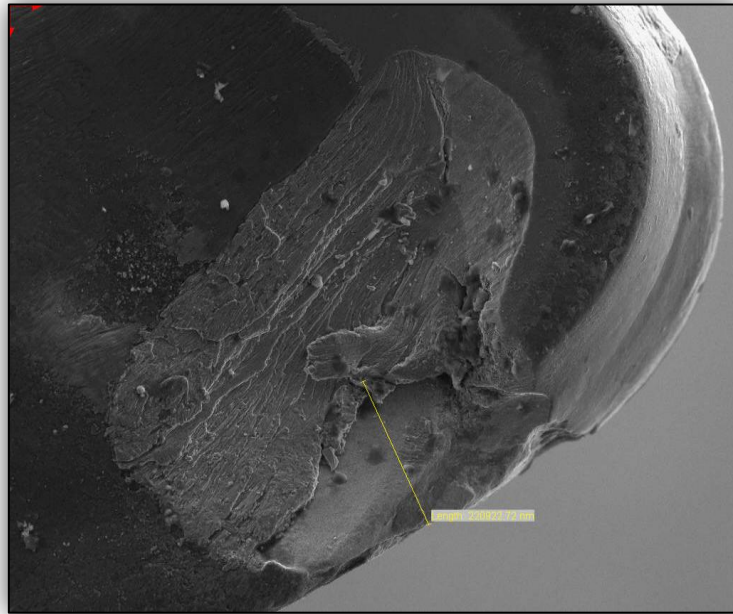
Figura 4.2 AGRIETAMIENTO EN EL FILO 1 DEL INSERTO 2.
