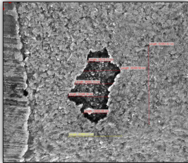
Figura 2.12 DETALLE DE LA FISURA EN LA TERCERA PASADA CON UN AUMENTO DE 2000X.
