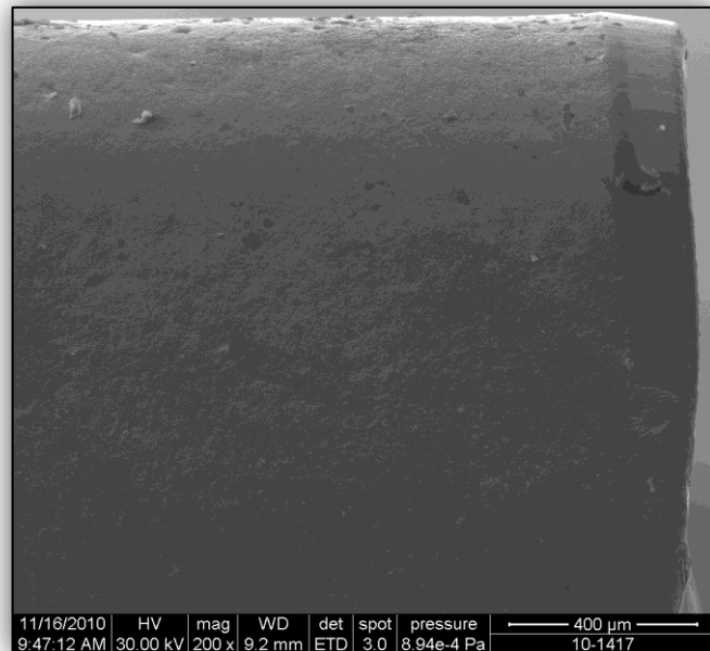
Figura 2.9 FILO # 5 EN LA SEGUNDA PASADA CON UN AUMENTO DE 200X.
