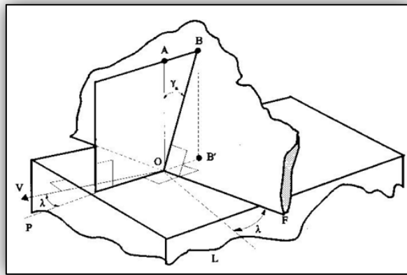
Figura 1.1 MODELO DE CORTE OBLICUO
