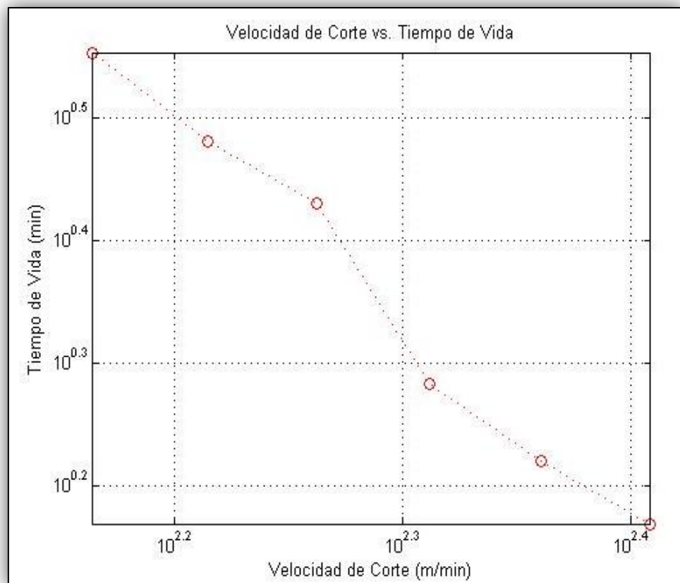
Gráfica 3.1 VELOCIDAD DE CORTE VS. TIEMPO DE MECANIZACIÓN (RELACIÓN DE TAYLOR) PARA INSERTO 1
