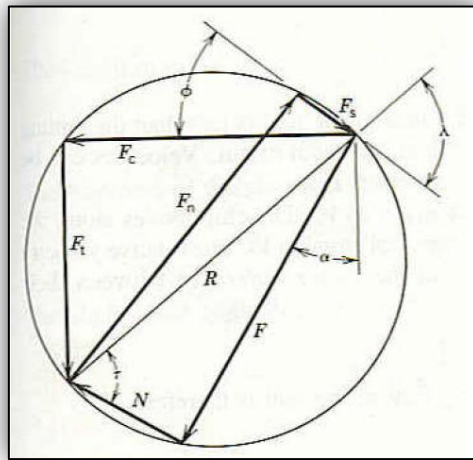
Figura 1.7 RELACIÓN ENTRE LAS FUERZAS DE CORTE.
