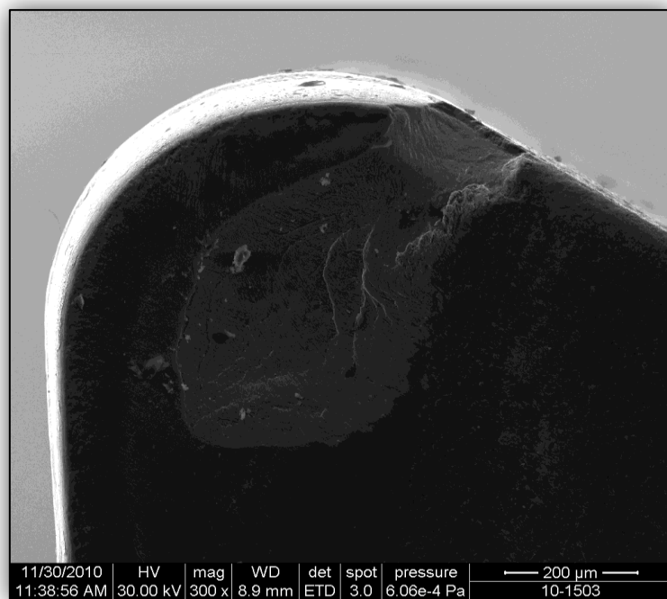
Figura 4.3 AGRIETAMIENTO EN EL FILO 2 DEL INSERTO 2.
