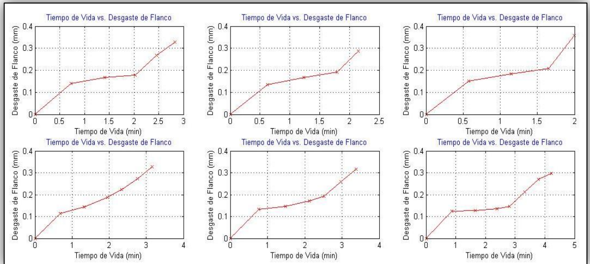
Gráfica 3.16 DESGASTE DE FLACO VS. TIEMPO DE VIDA PARA CADA UNO DE LOS FILOS DE CORTE DEL INSERTO 2 (VER APÉNDICE F)
