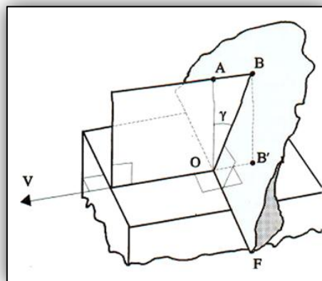
Figura 1.2 MODELO DE CORTE ORTOGONAL.
