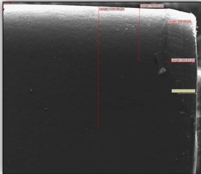
Figura 2.6 MEDICIÓN DEL DESGASTE DE FLANCO.
