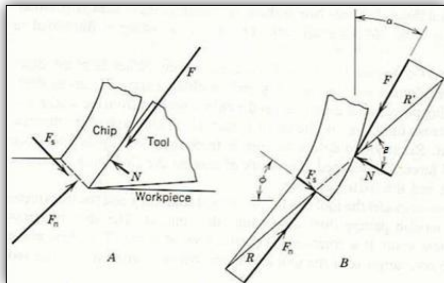
Figura 1.5 DIAGRAMA DE CUERPO LIBRE DE LA VIRUTA.
