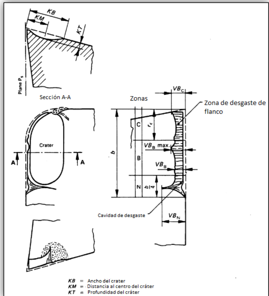
Figura 2.4 ZONAS DE DESGASTE DE LA HERRAMIENTA.
