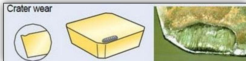
Figura 1.9 DESGASTE DE CRÁTER.
