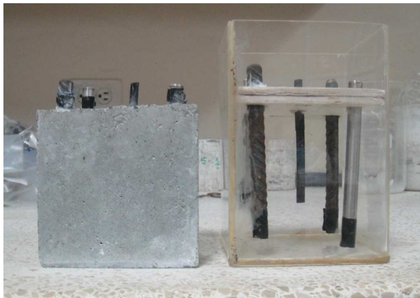
FIGURA 2.3 CELDA CONSTRUIDA CON LAS MISMAS PROPIEDADES QUE LAS DE HORMIGÓN
