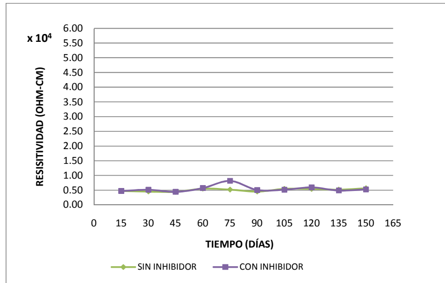
FIGURA 3.11 HORMIGÓN PUZOLÁNICO, INMERSAS EN CLORURO DE SODIO
