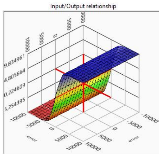
Figura 156. Representación gráfica de la superficie de salida
