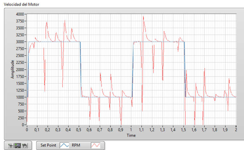
Figura 12. Respuesta de la planta con Control PID Convencional con perturbación
