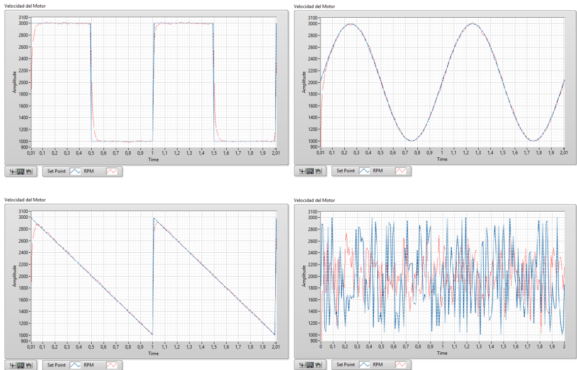
Figura 10. Respuesta del Sistema a Controlador PI Convencional
