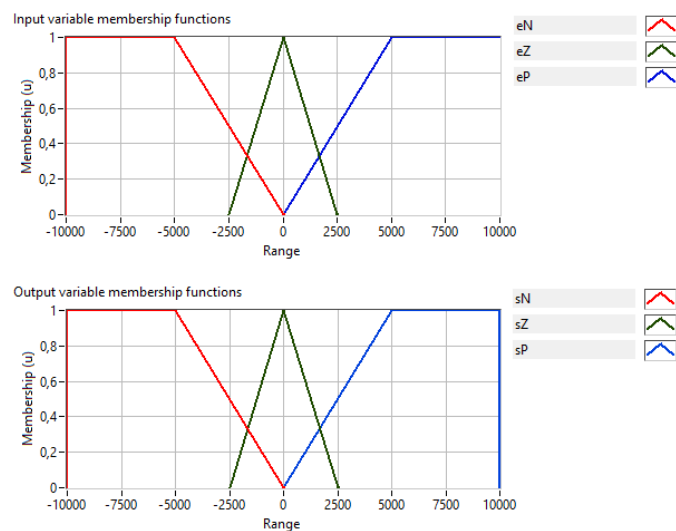
Figura 134. Diseño del Sistema Difuso con LabVIEW
