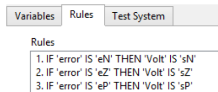
Figura 145. Reglas difusas para el Controlador Fuzzy
