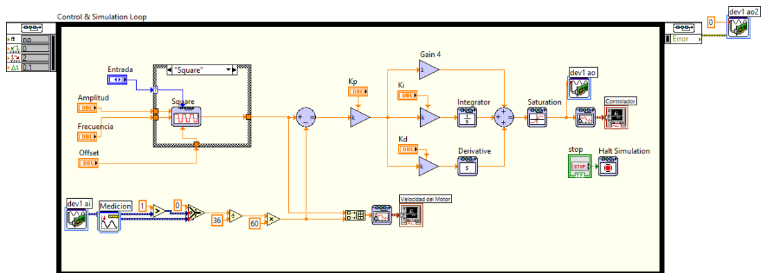
Figura 6. Diagrama de Bloques para Control de Velocidad PID de un Motor DC
