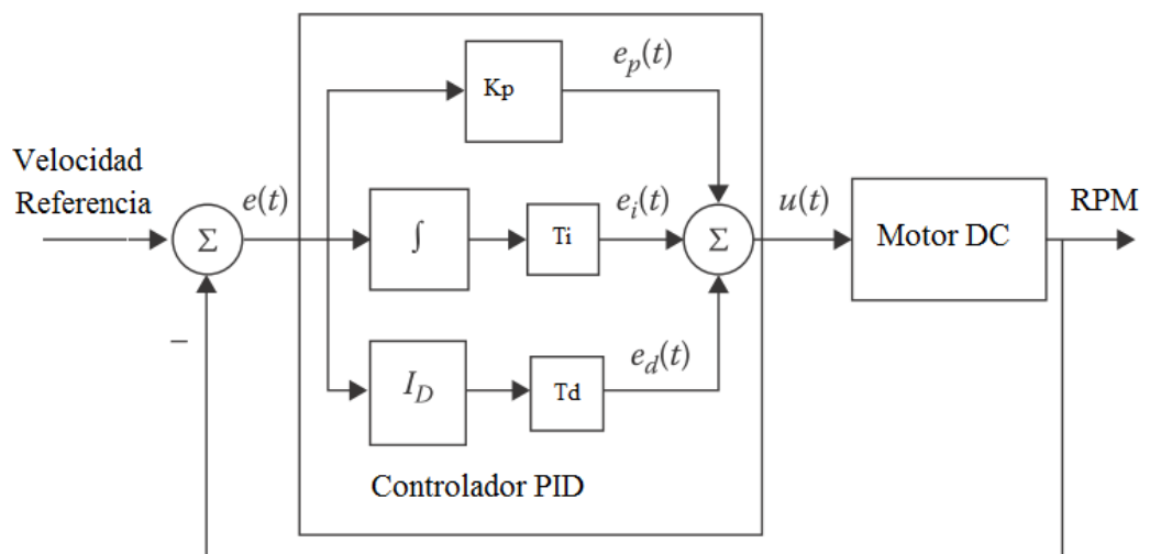
Figura 5. Diagrama de Bloques del Controlador PID Convencional
