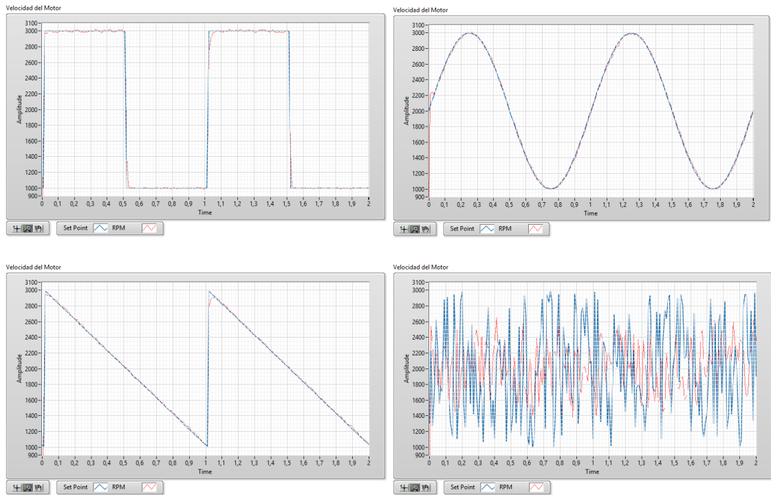
Figura 201. Respuesta del Sistema a Controlador Fuzzy PID
