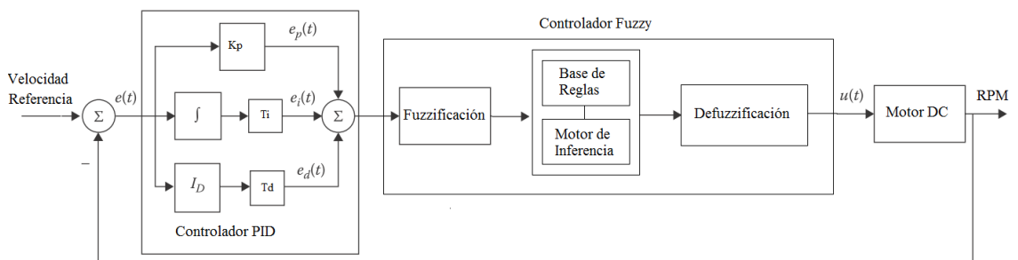
Figura 12. Digrama de Bloques de Controlador PID + Fuzzy
