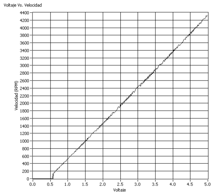
Figura 3. Respuesta de Velocidad del Motor DC
