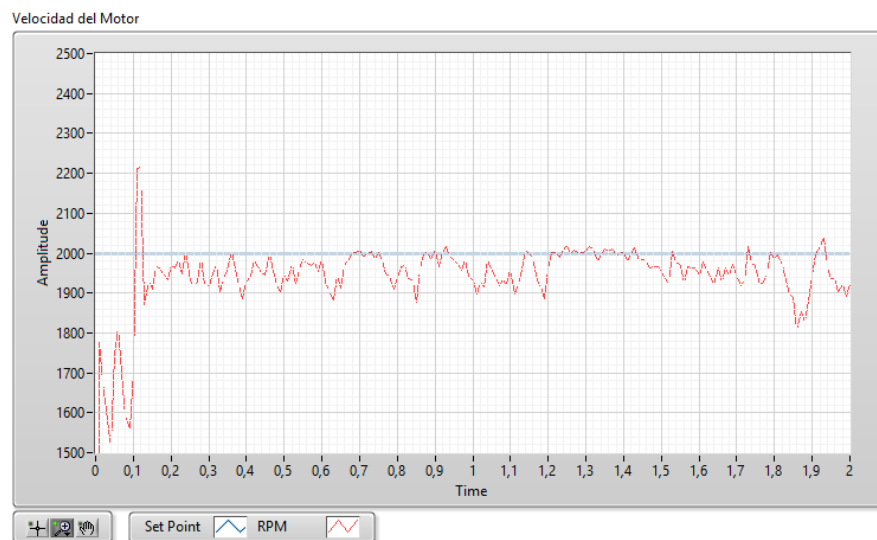
Figura 7. Respuesta del Sistema para K_p crítico
