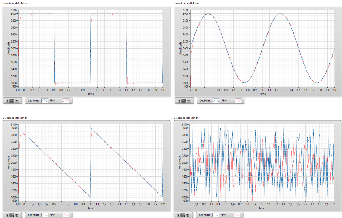
Figura 11. Respuesta del Sistema a Controlador PID Convencional
