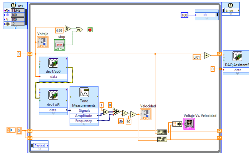
Figura 4. Caracterización del Motor DC
