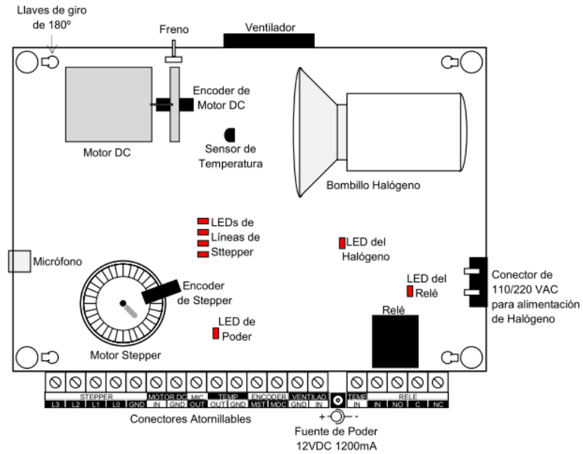
Figura 1. Diagrama Esquemático de la Planta EPC
