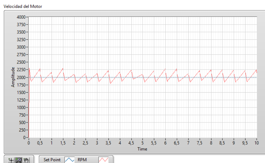
Figura 178. Respuesta del Sistema para K p crítico en controlador Fuzzy
