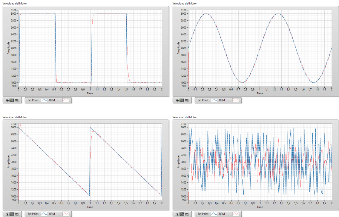
Figura 19. Respuesta del Sistema a Controlador Fuzzy PI
