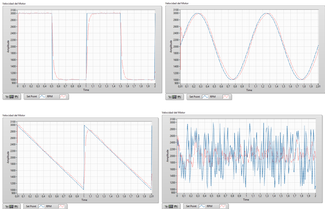
Figura 189. Respuesta del Sistema a Controlador Fuzzy P
