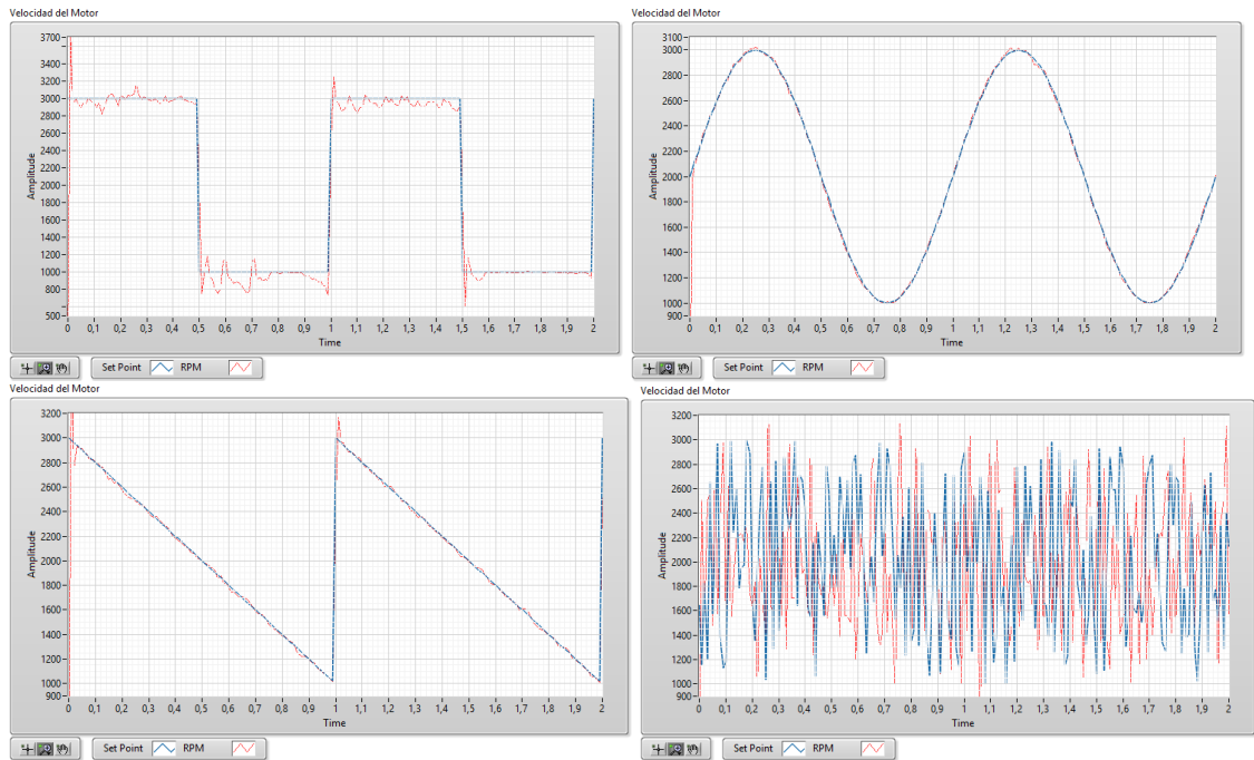
Figura 9. Respuestas del Sistema para Controlador P Convencional
