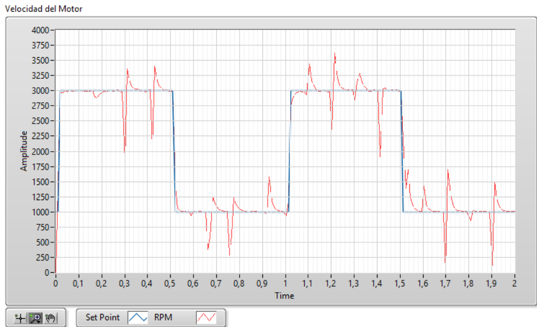
Figura 22. Respuesta de la planta con Control Fuzzy PID con perturbación
