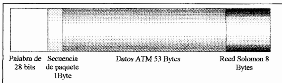
Figura 4.21. Estructura de un frame de datos de subida
