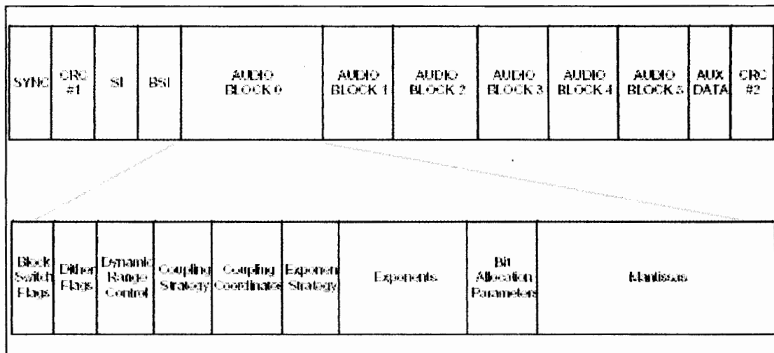
Figura 3.3. Frame de audio AC-3
