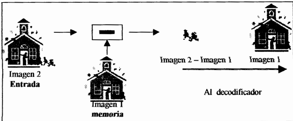
Figura 2.7. Predicción Interframe
