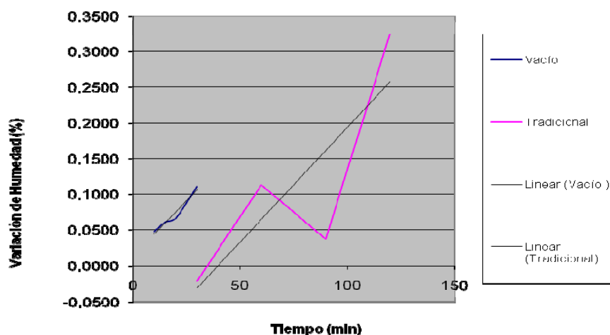
FIGURA 3.3 VARIACIÓN DE HUMEDAD VS TIEMPO EN LOS PROCESOS DE IMPREGNACIÓN AL VACÍO Y TRADICIONAL
