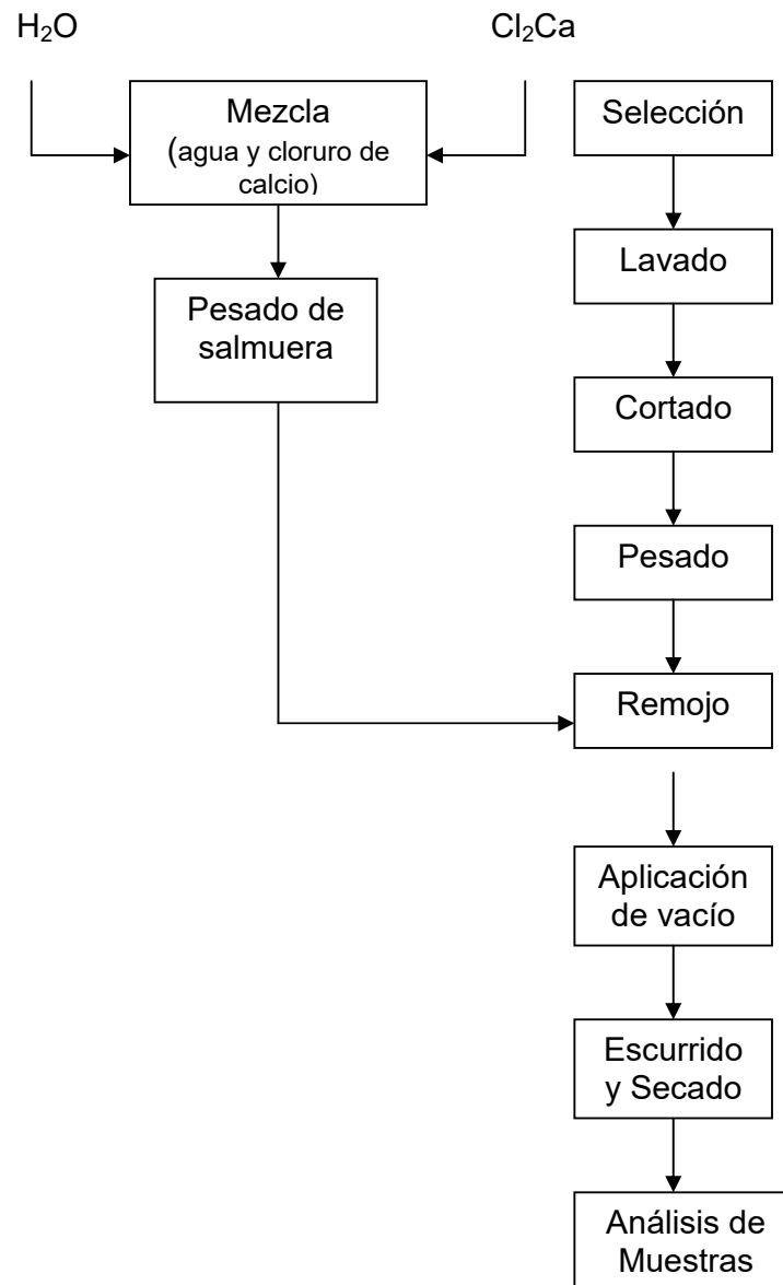
FIGURA 2.1 DIAGRAMA DE IMPREGNACIÓN DE CLORURO DE CALCIO POR MEDIO DE VACÍO EN REBANADAS DE PIMIENTO
