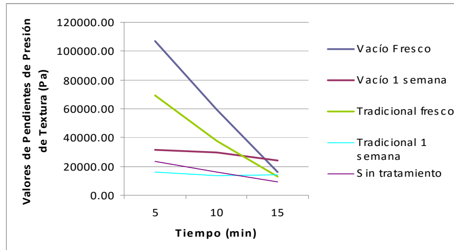
FIGURA 3.7 VALORES DE PENDIENTES DE LA PRESIÓN DE TEXTURA VS TIEMPO DE PROCESO TERMICO PARA LOS DISTINTOS TRATAMIENTOS
