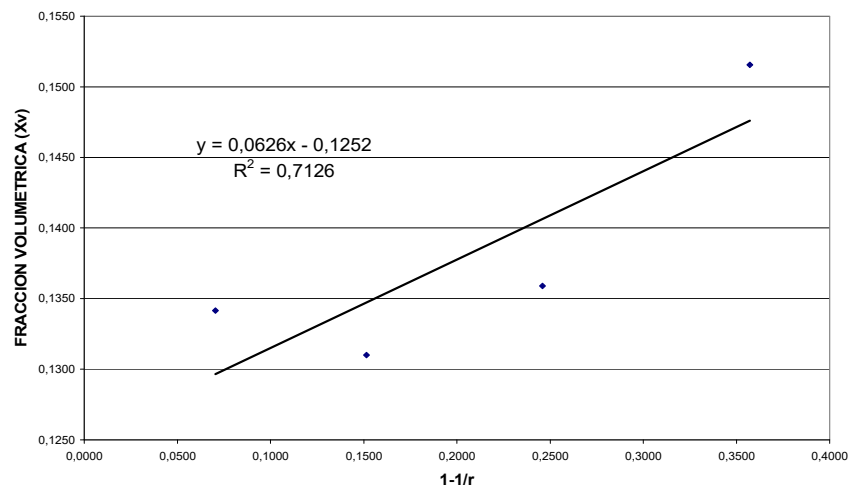
FIGURA 3.8 GRAFICO DE X VS 1-1/R PARA LOS EXPERIMENTOS REALIZADOS A DIFERENTES PRESIONES EN PIMIENTOS
