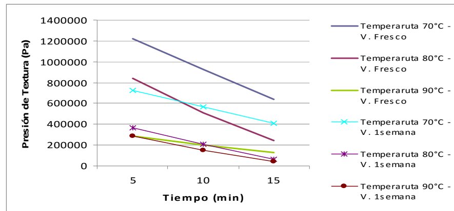
FIGURA 3.4 PRESIÓN DE TEXTURA VS TIEMPO DE TRATAMIENTO TERMICO PARA PIMIENTOS IMPREGNADOS AL VACÍO
