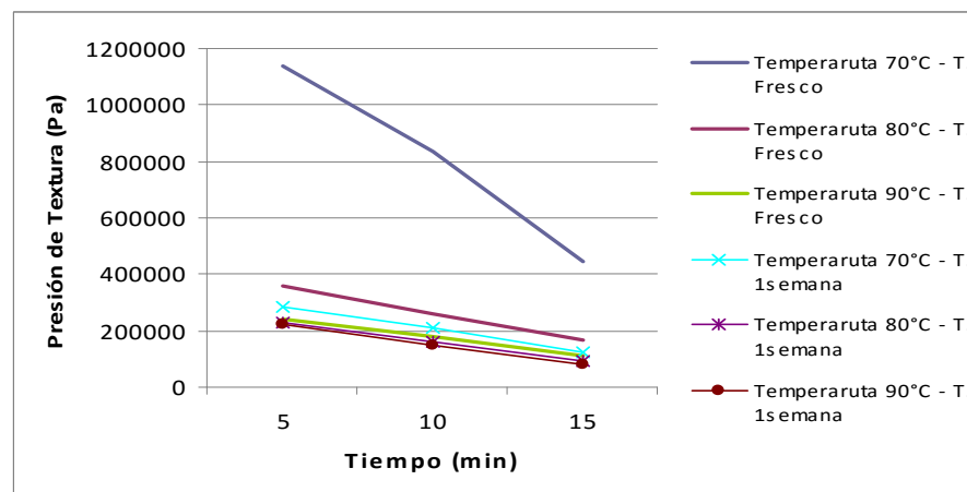
FIGURA 3.5 PRESIÓN DE TEXTURA VS TIEMPO DE TRATAMIENTO TERMICO PARA PIMIENTOS IMPREGNADOS TRADICIONALMENTE
