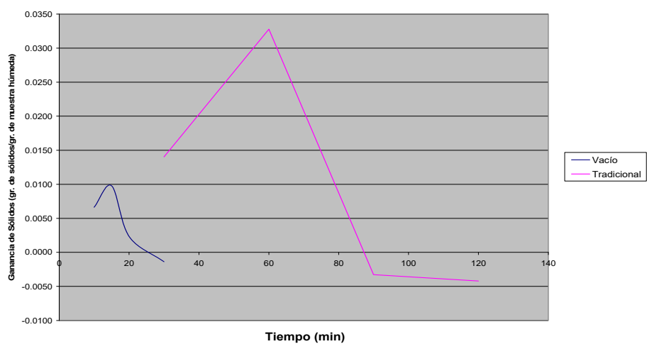
FIGURA 3.2 GANANCIA DE SÓLIDOS VS TIEMPO EN LOS PROCESOS DE IMPREGNACIÓN AL VACÍO Y TRADICIONAL
