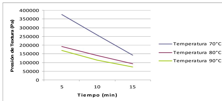
FIGURA 3.6 PRESIÓN DE TEXTURA VS TIEMPO DE TRATAMIENTO TERMICO PARA PIMIENTOS FRESCO SIN PROCESAR
