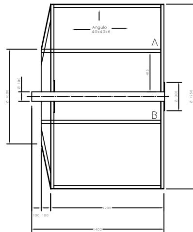
CORTE M-M
