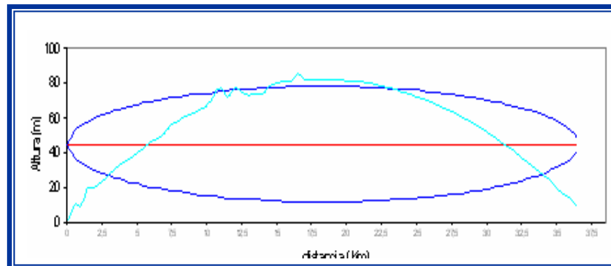
Fig. 55 Primera zonal de Fresnel de La Chivería – La Cadena
