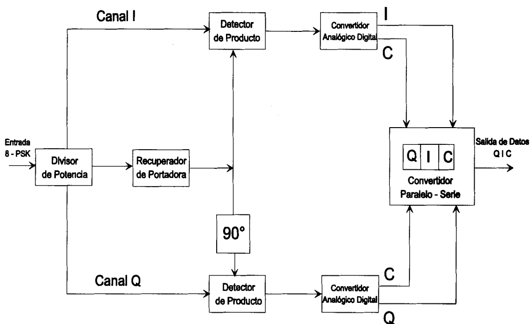
Demodulador 8 – PSK
