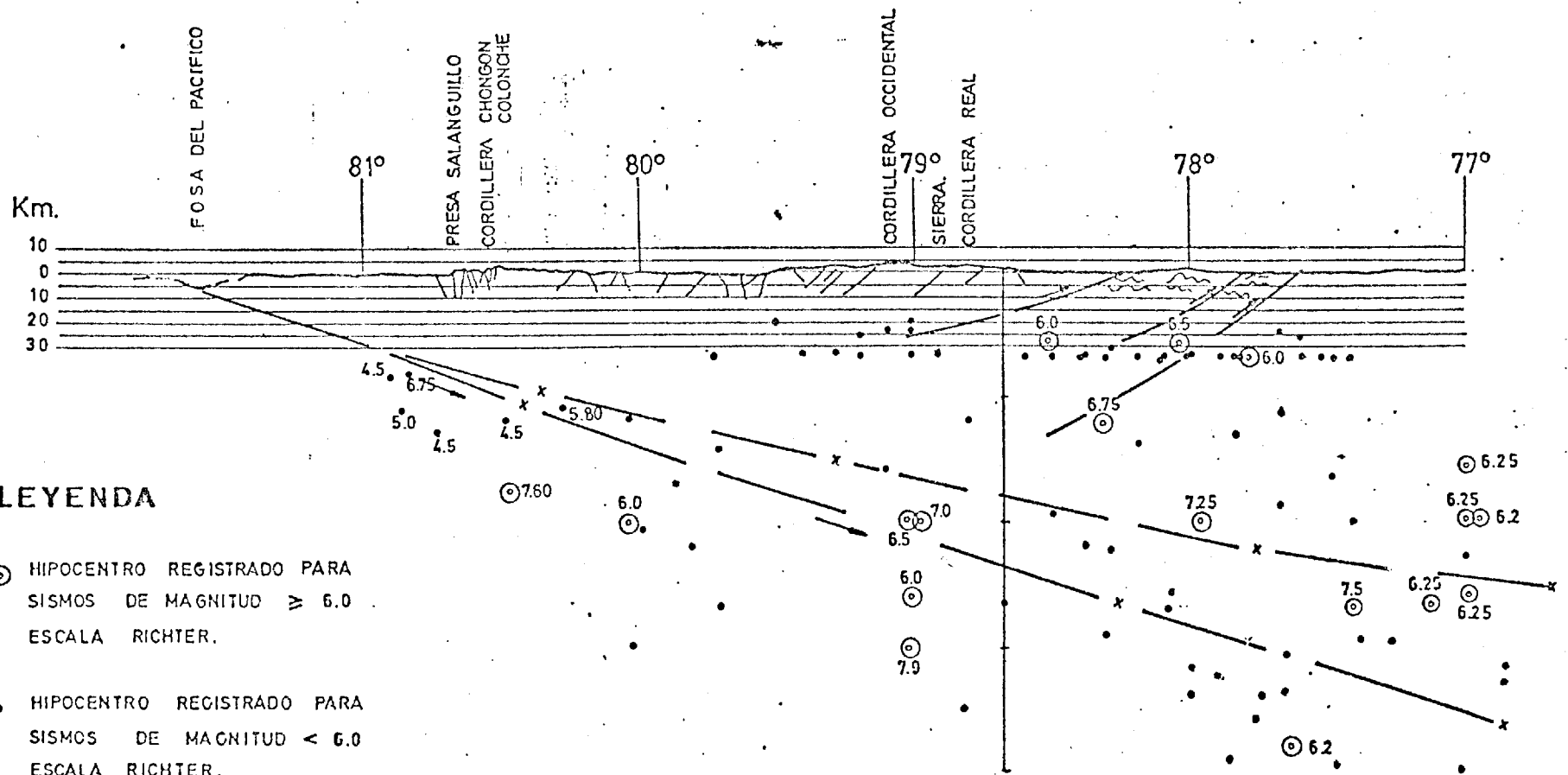
SECCION SISMICA
