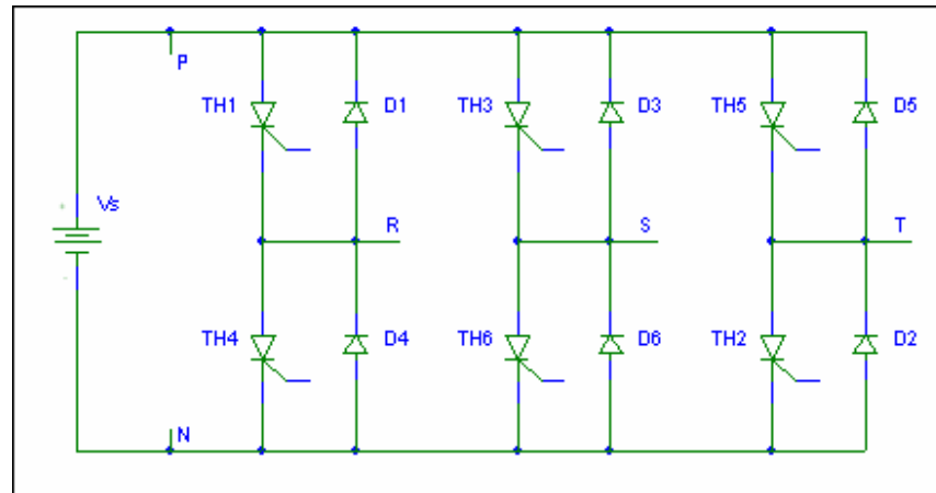
Fig. 2.5 Inversor trifásico.
